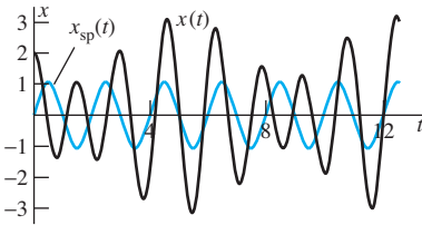
FIGURA 9.4.4. Solución periódica estacionaria x_{sp}(t) y la solución no periódica x(t) .
