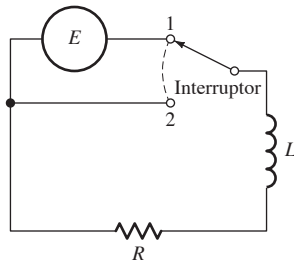
FIGURA 3.7.7. Circuito para los problemas 1 al 6.
