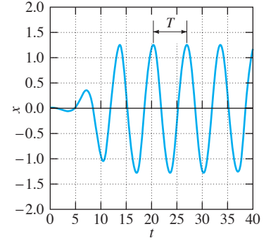
FIGURA 6.4.16. Curva solución en el plano tx con condiciones iniciales x(0) = 0.01 , x'(0) = 0 .
