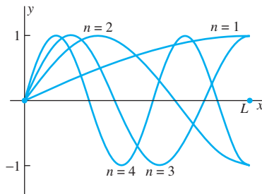
FIGURA 3.8.5. Las eigenfunciones y_n(x) = \sin \frac{(2n-1)\pi x}{2L} para n = 1, 2, 3, 4 .
