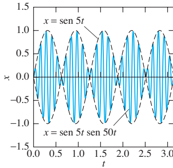
FIGURA 3.6.3. Fenómeno de las pulsaciones.
