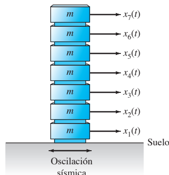
FIGURA 5.3.15. Edificio de siete pisos.
