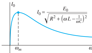
FIGURA 3.7.6. Efectos de la frecuencia en I_0 .
