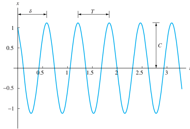
FIGURA 3.4.6. Gráfica de la función de la posición x(t) = C \cos(\omega_0 t - \alpha) en el ejemplo 1, con amplitud C \approx 1.118 , periodo T \approx 0.628 , y tiempo de retardo \delta \approx 0.582 .
