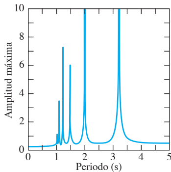
FIGURA 5.3.18. Vibraciones de resonancia de un edificio de siete pisos con amplitud máxima como una función del periodo.
