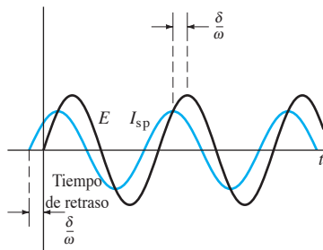
FIGURA 3.7.5. Tiempo de retraso de la corriente ocasionado por el voltaje suministrado.
