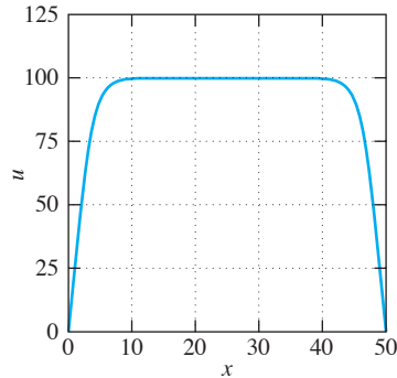
FIGURA 9.5.7. Gráfica de u(x, 30) que proporciona las temperaturas de la barra después de 30 s.
