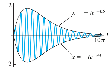
FIGURA 7.3.5 Gráfica de la oscilación amortiguada del problema 40.
