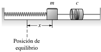
FIGURA 3.4.1. Sistema masa-resorte-amortiguador.
