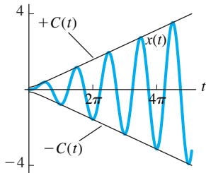
FIGURA 7.3.4. La solución de resonancia en (18) con \omega_0 = \frac{1}{2} y F_0 = 1 junto con sus curvas envolventes x = \pm C(t) .
