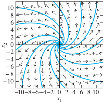
FIGURA 5.2.4. Campo direccional y curvas solución para el sistema lineal x'_1 = 4x_1 - 3x_2 , x'_2 = 3x_1 + 4x_2 del ejemplo 3.
