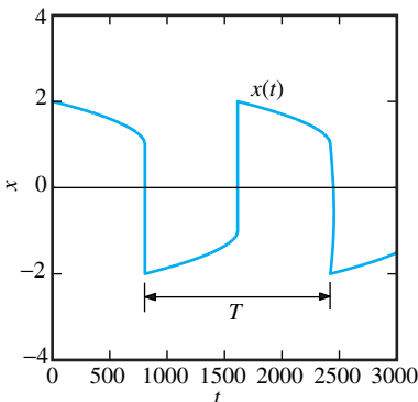
FIGURA 6.4.21. Gráfica de x(t) con \mu = 1000 .
