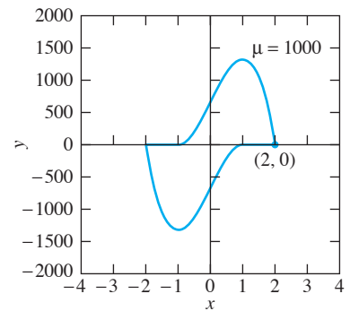
FIGURA 6.4.20. Trayectoria del plano de fase de la solución periódica de la ecuación de van der Pol con \mu = 1000 .
