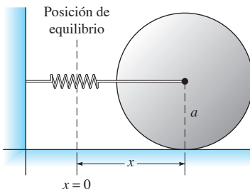
FIGURA 3.6.5. El disco rodando.
