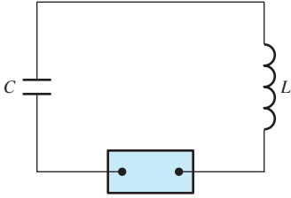
FIGURA 6.4.17. Circuito simple con un elemento activo.
