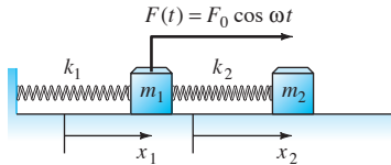
FIGURA 5.3.12. Sistema mecánico del problema 14.
