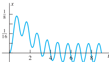
FIGURA 7.5.18. Respuesta x(t) a la excitación de entrada de una onda cuadrada con periodo 1.
