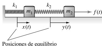
FIGURA 4.1.1. Sistema masa-resorte del ejemplo 1.
