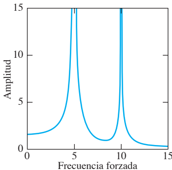
FIGURA 5.3.10. Gráfica de frecuencia-amplitud para el ejemplo 3.
