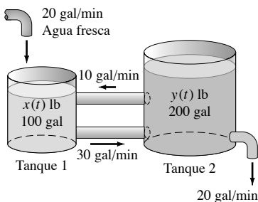
FIGURA 4.1.3. Los dos tanques de salmuera del ejemplo 2.
