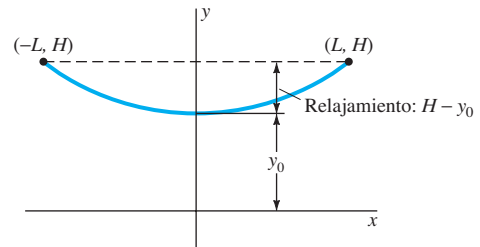
FIGURA 1.4.12. La catenaria.
