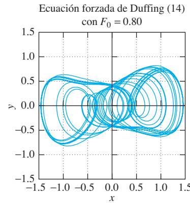
FIGURA 6.5.16(a). Respuesta caótica con F_0 = 0.80 : trayectoria del plano de fase.
