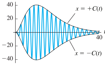
FIGURA 7.3.6. La solución de resonancia y sus curvas envolventes en el caso 4.
