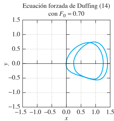
FIGURA 6.5.14(a). Respuesta de periodo 4\pi con F_0 = 0.70 : trayectoria del plano de fase.
