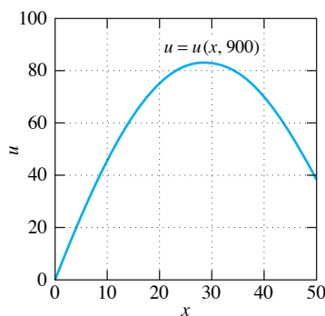
FIGURA 10.2.7. Temperaturas en la lámina después de 15 min.
