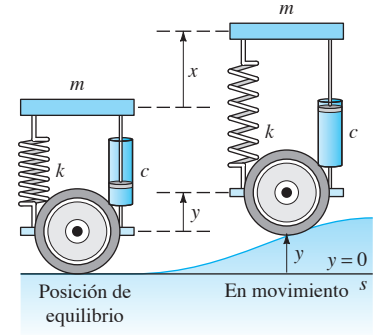
FIGURA 3.6.7. “Modelo monociclo” de un carro.
