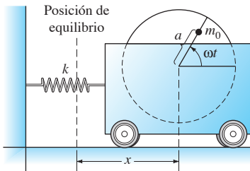
FIGURA 3.6.1. Sistema de la carreta con volante.
