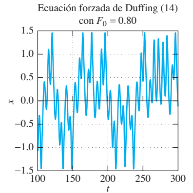
FIGURA 6.5.16(b). Respuesta caótica con F_0 = 0.80 : solución x(t) .
