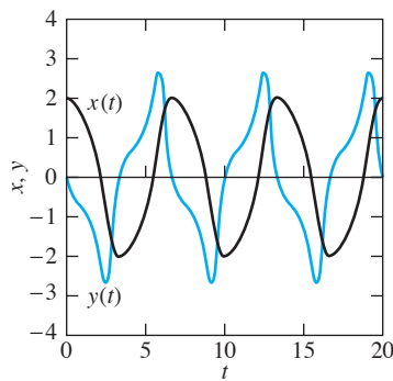
FIGURA 6.4.19. Curvas solución x(t) y y(t) que definen la solución periódica de la ecuación de van der Pol con \mu = 1 .
