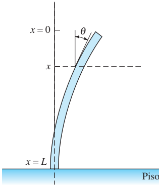
FIGURA 8.6.1. Pandeo de la columna.
