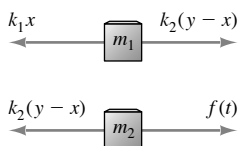
FIGURA 4.1.2. “Diagramas de cuerpo libre” para el sistema del ejemplo 1.
