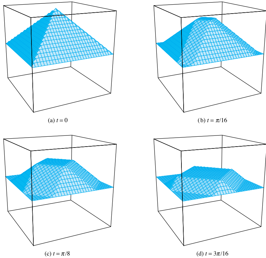
FIGURA 10.5.3. Vibraciones de la membrana cuadrada con periodo P = \pi\sqrt{2} .
