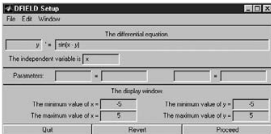
FIGURA 1.3.29. Menú de inicio de MATLAB dfield para construir el campo de isoclinas y las curvas solución para y' = \sin(x - y) .
