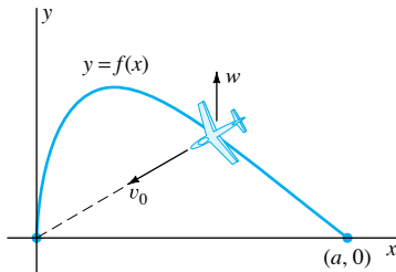
FIGURA 1.6.4. El avión se dirige al origen.
