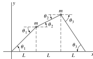
FIGURA 4.1.12. Sistema mecánico del problema 25.
