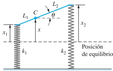
FIGURA 5.3.14. Modelo de un automóvil con dos ejes.
