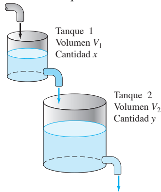
FIGURA 1.5.5. Cascada de dos tanques.
