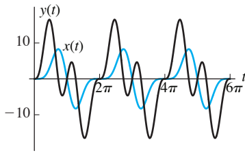
FIGURA 7.2.6. Funciones de la posición x(t) y y(t) del ejemplo 3.
