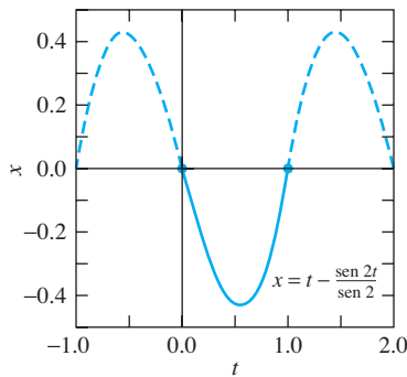
FIGURA 9.3.6. Gráfica de la solución del ejemplo 2.
