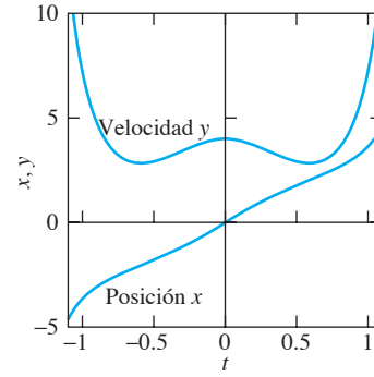
FIGURA 6.4.5. Curvas solución de posición y velocidad para el sistema masa y resorte suave con m = 1 , k = 4 y \beta = 1 > 0 y energía E = 8 —suficientemente grande para que la masa se aproxime al origen desde la izquierda y continúe indefinidamente hacia la derecha.
