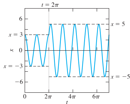
FIGURA 7.6.3. Movimiento de la masa en el ejemplo 1.
