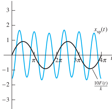
FIGURA 9.4.7. Fuerza impuesta y movimiento periódico estacionario resultante del ejemplo 4.
