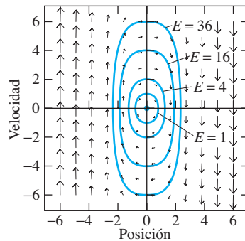
FIGURA 6.4.2. Plano de fase posición-velocidad para el sistema masa-resorte duro con m = k = 2 y \beta = -4 < 0 .
