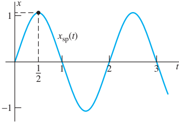
FIGURA 9.4.3. Gráfica de la solución periódica estacionaria x_{sp}(t) .
