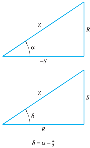
FIGURA 3.7.4. Reactancia y ángulo de retraso.
