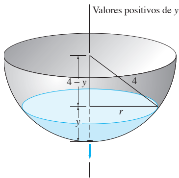
FIGURA 1.4.9. Drenado de un tanque semiesférico.
