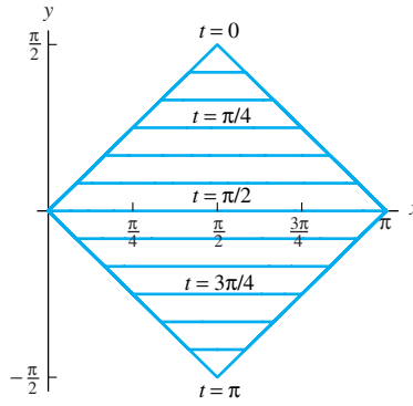
FIGURA 9.6.6. Posiciones sucesivas de la cuerda vibrando con posición inicial triangular.
