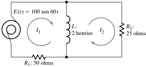
FIGURA 4.1.14. Circuito eléctrico del problema 27.
