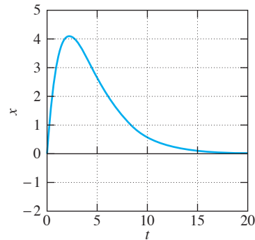
FIGURA 3.4.14. Función de la posición x(t) del problema 13.
