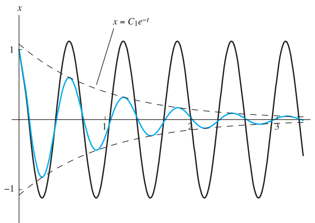
FIGURA 3.4.10. Gráficas de la función de la posición x(t) = C_1 e^{-t} \cos(\omega_1 t - \alpha_1) del ejemplo 2 (oscilaciones amortiguadas), la función de la posición x(t) = C \cos(\omega_0 t - \alpha) del ejemplo 1 (oscilaciones no amortiguadas) y las curvas envolventes x(t) = \pm C_1 e^{-t} .
