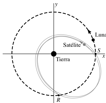
FIGURA 4.3.11. La Luna y el satélite en un sistema coordenado no giratorio 1.5 días después de la inserción orbital del satélite en el punto de inicio S .
