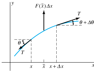
FIGURA 9.6.1. Fuerzas en un segmento pequeño de cuerda vibrando.
