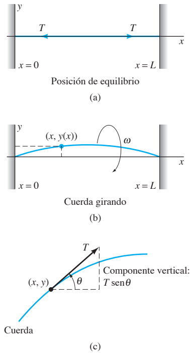
FIGURA 3.8.6. Cuerda girando.
