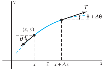
FIGURA 3.8.7. Fuerzas en un pequeño segmento de la cuerda girando.
