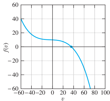
FIGURA 2.6.7. Gráfica de f(v) = 9.8 - (0.00016)(100v + 10v^2 + v^3) .
