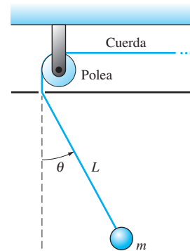
FIGURA 8.6.6. Péndulo de longitud variable.
