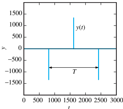
FIGURA 6.4.22. Gráfica de y(t) con \mu = 1000 .
