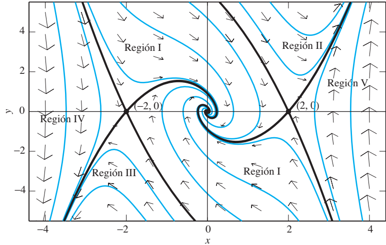
FIGURA 6.4.6. Plano de fase posición-velocidad para el sistema masa-resorte suave con m = 1 , k = 5 , \beta = \frac{5}{4} y constante de resistencia c = 2 . Las separatrices están resaltadas (marcadas en negro).
