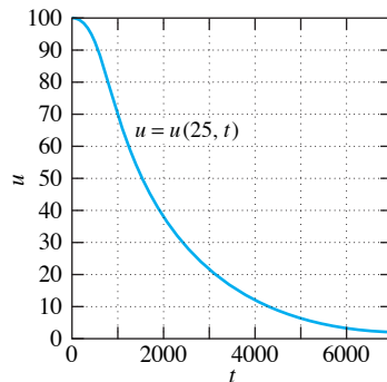
FIGURA 9.5.9. Gráfica de u(25, t) que proporciona la temperatura en el punto medio de la barra.
