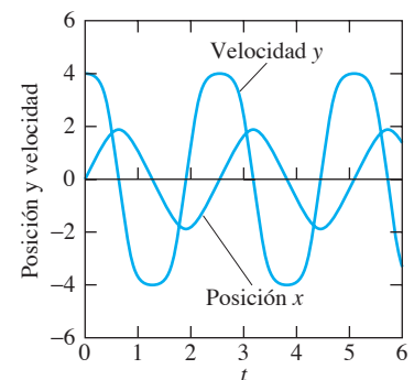
FIGURA 6.4.3. Curvas solución posición y velocidad para el sistema masa-resorte duro con m = k = 2 y \beta = -4 < 0 .
