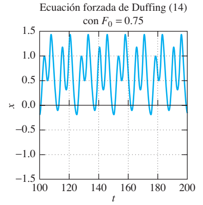
FIGURA 6.5.15(b). Respuesta de periodo 8\pi con F_0 = 0.75 : solución x(t) .
