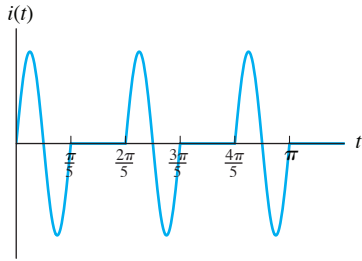
FIGURA 7.6.8. Función de la corriente del problema 20.
