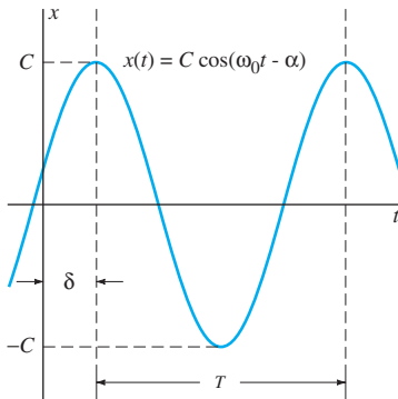
FIGURA 3.4.5. Movimiento armónico simple.
