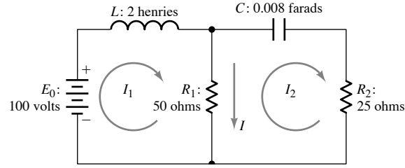
FIGURA 4.1.4. Red eléctrica del ejemplo 3.
