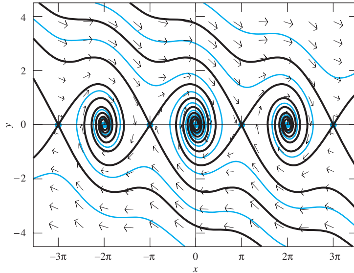
FIGURA 6.4.10. Plano de fase posición-velocidad para el sistema del péndulo amortiguado x' = y , y' = -\sin x - \frac{1}{4}y . Las separatrices están remarcadas (en negro).
