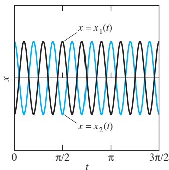
FIGURA 5.3.5. Oscilaciones en direcciones opuestas con frecuencia \omega_2 = 10 ; las amplitudes de movimiento de las dos masas son las mismas.
