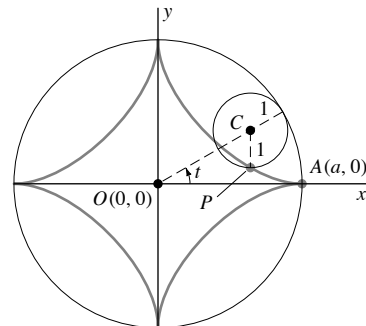
FIGURA 4.2.8. La hipocicloide del problema 48.
