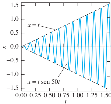
FIGURA 3.6.4. Fenómeno de resonancia.
