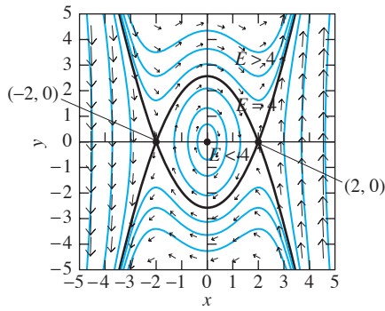
FIGURA 6.4.4. Plano de fase posición-velocidad para el sistema masa y resorte suave con m = 1 , k = 4 y \beta = 1 > 0 . Se marcan las separatrices (en negro).
