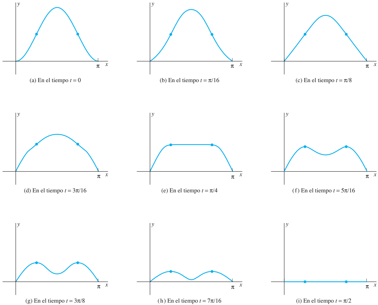
FIGURA 9.6.4. Fotografías instantáneas sucesivas de la cuerda vibrando de los problemas 23 y 24.
