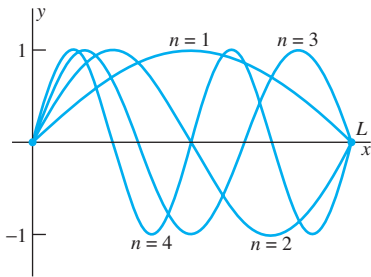
FIGURA 3.8.4. Eigenfunciones y_n(x) = \sin \frac{n\pi x}{L} para n = 1, 2, 3, 4 .
