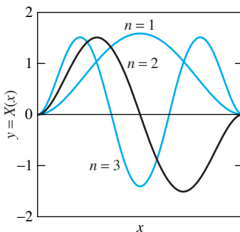
FIGURA 10.3.7. Primeras tres gráficas de la eigenfunción y = X_n(x) para la barra de sección I fija-fija.
