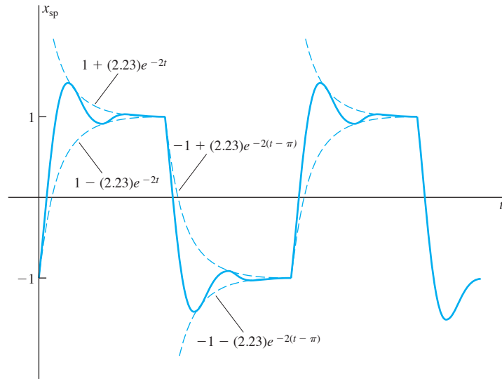
FIGURA 7.5.12. Gráfica de la solución periódica en estado permanente del ejemplo 8; nótese las oscilaciones “periódicamente amortiguadas” con una frecuencia cuatro veces mayor a la de la fuerza de excitación.
