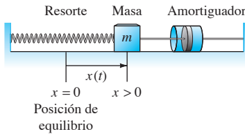
FIGURA 3.1.1. Sistema masa-resorte-amortiguador.
