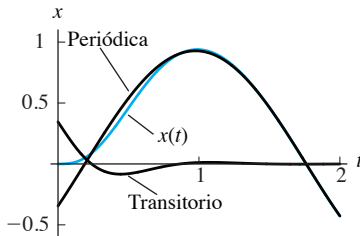
FIGURA 7.3.3. Oscilación periódica forzada x_{sp}(t) , movimiento transitorio amortiguado x_{tr}(t) y solución x(t) = x_{sp}(t) + x_{tr}(t) del ejemplo 4.
