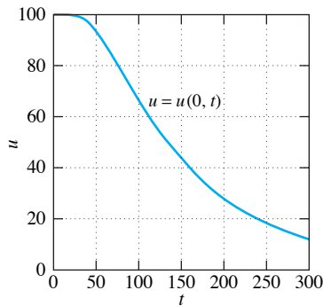
FIGURA 10.4.12. Temperatura de la línea central como función del tiempo t .
