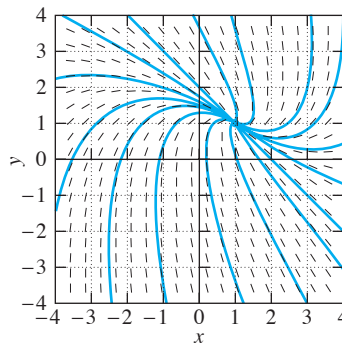
FIGURA 6.1.16. Nodo (1, 1) .
