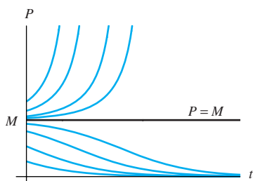
FIGURA 2.1.6. Curvas solución típicas para la ecuación explosión/extinción P' = kP(P - M) .
