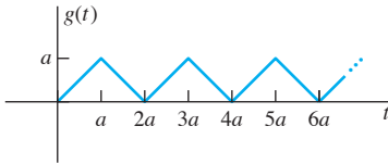
FIGURA 7.5.10. Gráfica de la función de onda triangular del ejemplo 7.
