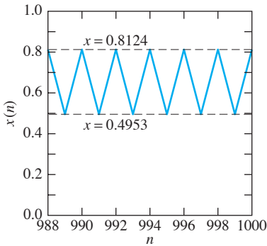
FIGURA 6.5.4. Gráfica de x(n) = x_n , mostrando el ciclo de periodo 2 de las iteraciones obtenidas con r = 3.25 .
