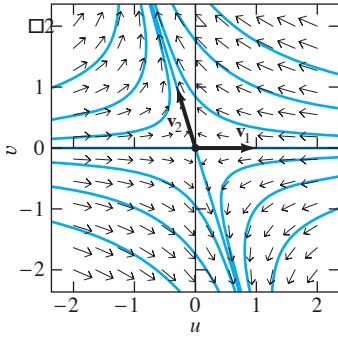
FIGURA 6.3.11. Plano de fase del sistema lineal de la ecuación (22) correspondiente al punto crítico (7, 0) .
