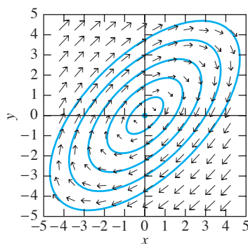
FIGURA 6.2.8. El centro estable del ejemplo 6.
