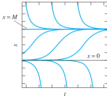
FIGURA 2.2.3. Curvas solución típicas para la ecuación logística dx/dt = kx(M - x) .
