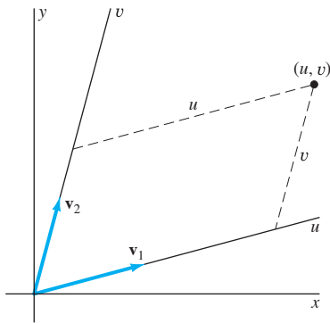
FIGURA 6.2.3. Sistema de coordenadas oblicuas uv determinado por los eigenvectores \mathbf{v}_1 y \mathbf{v}_2 .
