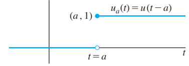
FIGURA 7.1.5. La función escalón unitario u_a(t) tiene un salto en t = a .
