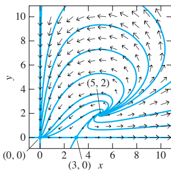
FIGURA 6.3.17. Caso en que \epsilon = -1 (problemas 20 a 22).
