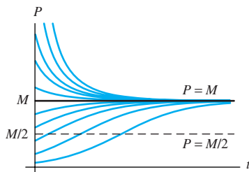
FIGURA 2.1.3. Curvas solución típicas para la ecuación logística P' = kP(M - P) . Cada curva solución que inicia debajo de la línea P = M/2 cuenta con un punto de inflexión. (Véase el problema 34.)
