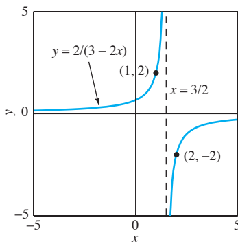
FIGURA 1.1.7. Solución de y' = y^2 definida por y(x) = 2/(3 - 2x) .
