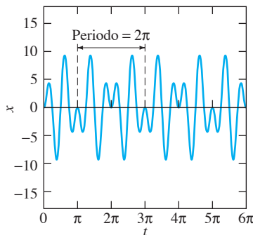
FIGURA 3.6.2. Respuesta x(t) = 5 \cos 3t - 5 \cos 5t del ejemplo 1.
