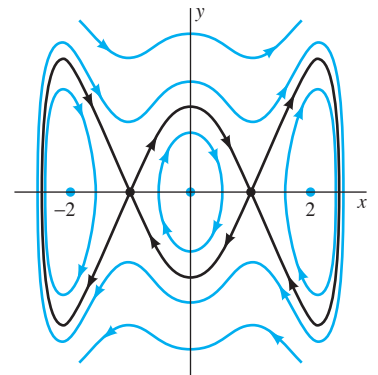
FIGURA 6.4.14. Plano de fase del problema 16.
