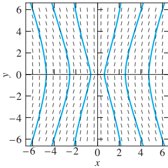
FIGURA 1.6.2. Campo de isoclinas y curvas solución para 2xyy' = 4x^2 + 3y^2 .
