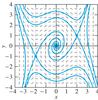
FIGURA 6.1.15. Punto espiral (0, 0) ; punto silla (-2, -1) y (2, 1) .
