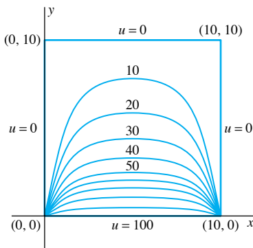
FIGURA 9.7.4. Curvas de nivel típicas de la función u(x, y) en la ecuación (15).
