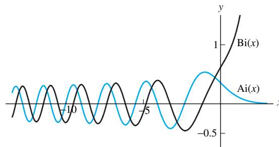
FIGURA 8.2.3. Gráficas de la función de Airy y = \text{Ai}(x) y y = \text{Bi}(x) .
