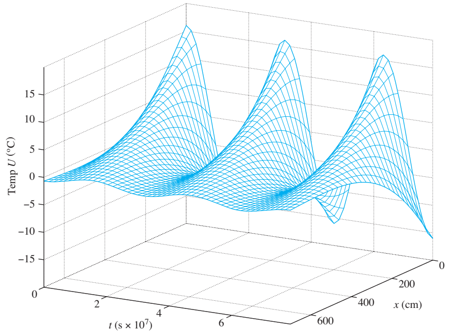
FIGURA 10.3.4. Gráfica de la función de temperatura U(x, t) de la ecuación (29).
