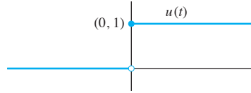
FIGURA 7.1.4. Gráfica de la función escalón unitario.
