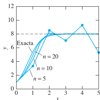
FIGURA 2.4.9. Aproximación a una solución logística utilizando el método de Euler con n = 5 , n = 10 y n = 20 subintervalos.
