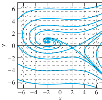
FIGURA 6.1.18. Punto espiral (-2, \frac{2}{3}) y punto silla (2, -\frac{2}{5}) .
