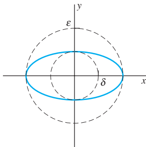
FIGURA 6.1.9. Si el punto inicial (x_0, y_0) se encuentra dentro de una distancia \delta del origen, entonces el punto (x(t), y(t)) permanece dentro de una distancia \epsilon del origen.
