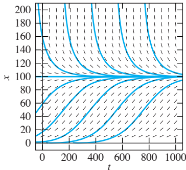
FIGURA 1.4.14. Campo de isoclinas y curvas solución para x' = (0.01)x - (0.0001)x^2 .
