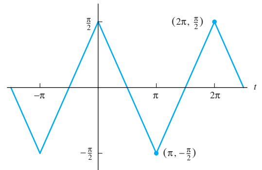
FIGURA 9.3.10. Función de onda triangular par de periodo 2\pi .
