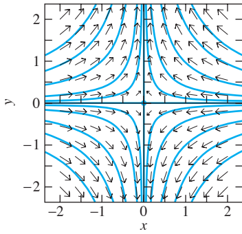
FIGURA 6.1.7. Punto silla cuyas trayectorias se asemejan al contorno de las curvas de un punto silla sobre una superficie.
