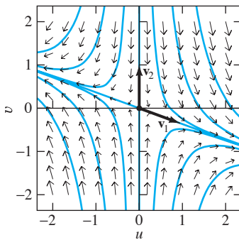
FIGURA 6.3.10. Plano de fase del sistema lineal de la ecuación (20) correspondiente al punto crítico (0, 8) .
