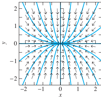
FIGURA 6.1.6. Nodo impropio: Todas las trayectorias son tangentes a una recta, se aproximan al origen, por tanto es un nodo convergente.
