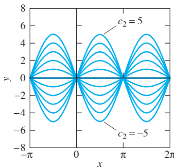
FIGURA 3.1.4. Soluciones y(x) = c_2 \sin x de y'' + y = 0 .
