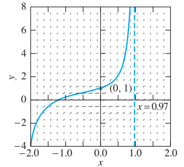
FIGURA 2.4.12. Solución de dy/dx = x^2 + y^2 , y(0) = 1 .
