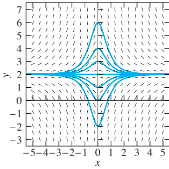
FIGURA 1.5.2. Campo de isoclinas y curvas solución para la ecuación diferencial de la ecuación (9).
