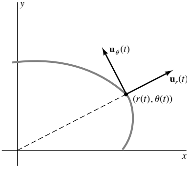
FIGURA 4.1.16. Vectores unitarios radial y transversal \mathbf{u}_r y \mathbf{u}_\theta .
