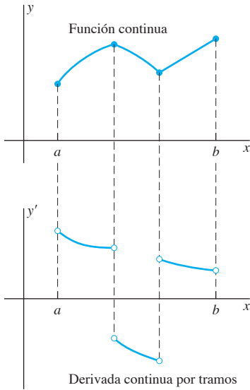
FIGURA 7.2.1. Discontinuidades de f' que corresponden a “esquinas” en la gráfica de f .
