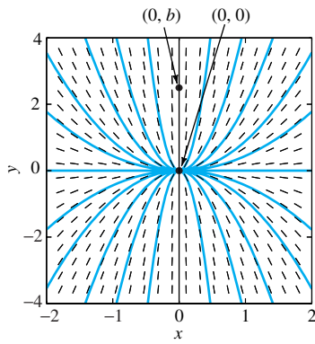
FIGURA 1.3.13. En el punto (0, 0) existe infinidad de curvas solución pero ninguna que pase por el punto (0, b) si b \neq 0 .
