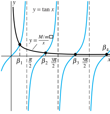
FIGURA 10.2.3. Raíces positivas \{\beta_n\}_1^\infty de la ecuación (22).
