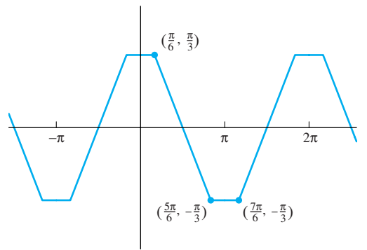
FIGURA 9.3.8. Función de onda trapezoidal par de periodo 2\pi .
