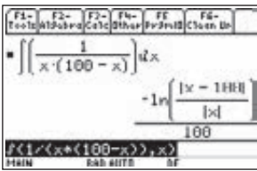
FIGURA 1.4.13. Pantalla de la TI-89 mostrando la integral de la ecuación (3).
