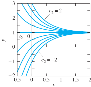
FIGURA 3.1.9. Soluciones y(x) = 1 + c_2 e^{-2x} de y'' + 2y' = 0 con diferentes valores de c_2 .
