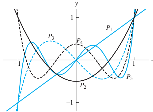
FIGURA 8.2.2. Gráficas de los polinomios de Legendre y = P_n(x) para n = 1, 2, 3, 4 y 5 . Las gráficas se caracterizan por el hecho de que todas las raíces de P_n(x) se encuentran en el intervalo -1 < x < 1 .
