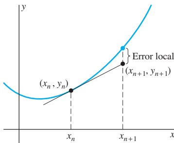
FIGURA 2.4.6. Error local del método de Euler.
