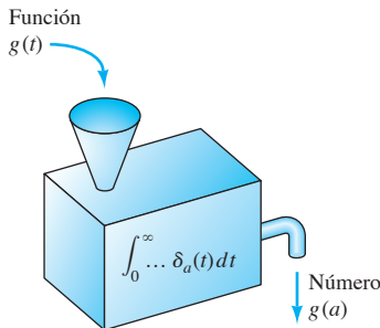
FIGURA 7.6.2. Diagrama que ilustra cómo la función delta “filtra” el valor g(a) .
