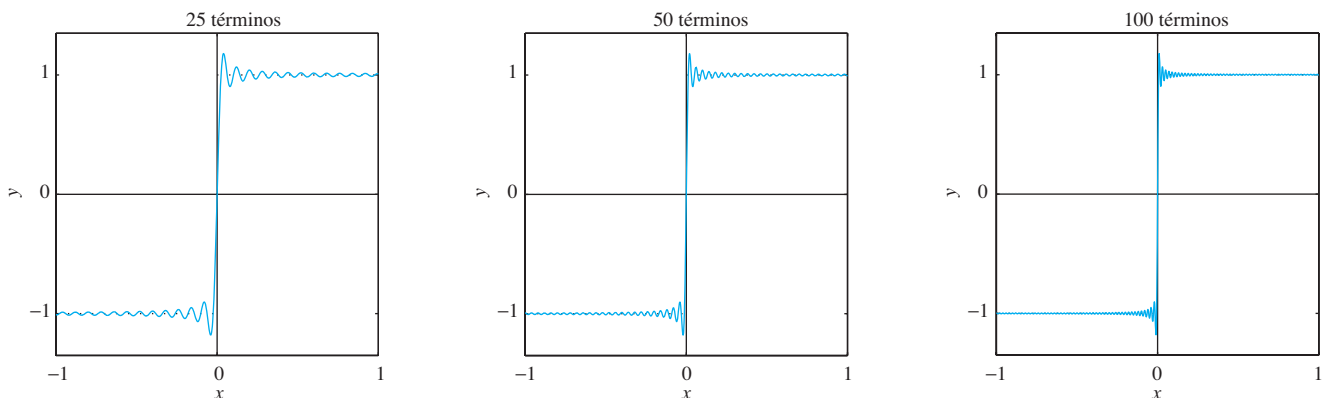
FIGURA 10.1.6. Gráficas con N = 25 , N = 50 , N = 100 de la suma parcial de \sum_{n=1}^N c_n \sin \beta_n x de la serie en términos de eigenfunciones de la ecuación (1).
