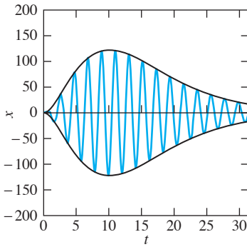
FIGURA 3.6.15. Solución x(t) = e^{-t/5}[3t \cos t + (9t^2 - 1) \sin 3t] y las curvas envolventes x(t) = \pm e^{-t/5} \sqrt{(3t)^2 + (9t^2 - 1)^2} con fuerza externa F(t) = 2700te^{-t/5} \cos 3t .
