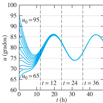
FIGURA 1.5.10. Curvas solución dadas por la ecuación (5) con u_0 = 65, 68, 71, \dots, 92, 95 .
