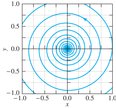
FIGURA 6.2.18 (d). Espiral inestable con \epsilon = 0.05 .
