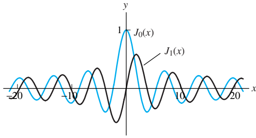
FIGURA 8.5.2. Gráficas de las funciones de Bessel J_0(x) y J_1(x) .
