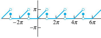
FIGURA 9.1.4. Función periódica del ejemplo 2.
