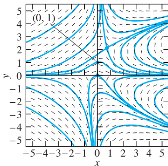
FIGURA 1.6.7. Campo de isoclinas y curvas solución para la ecuación exacta del ejemplo 9.
