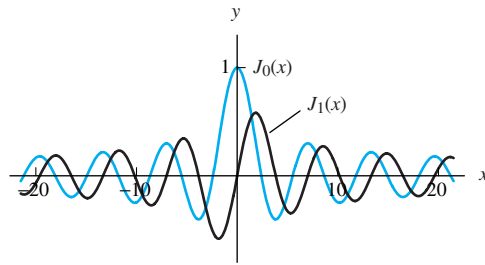
FIGURA 10.4.2. Gráficas de las funciones de Bessel J_0(x) y J_1(x) .
