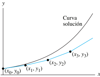
FIGURA 2.4.1. Primeros pequeños pasos para aproximar una curva solución.
