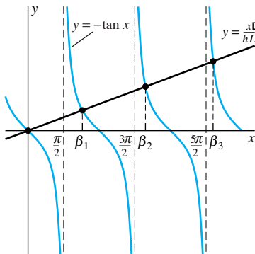
FIGURA 10.1.1. Solución de la ecuación (17) por métodos geométricos.
