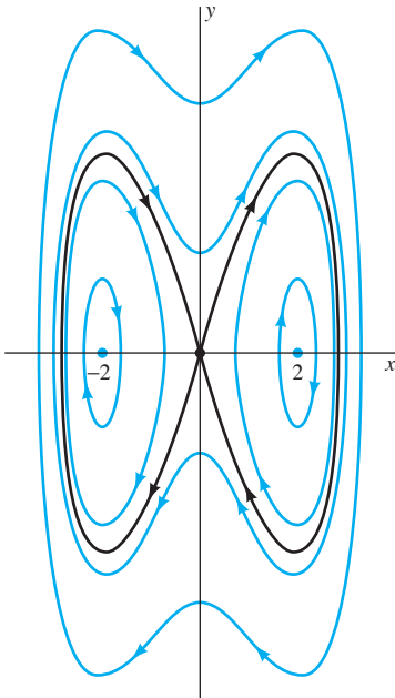
FIGURA 6.4.12. Plano de fase del problema 14.
