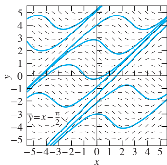
FIGURA 1.3.28. Campos de isoclinas y curvas solución generadas en computadora para la ecuación diferencial y' = \sin(x - y) .
