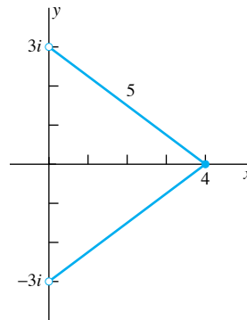
FIGURA 8.2.1. Radio de convergencia como la distancia a la singularidad más cercana.
