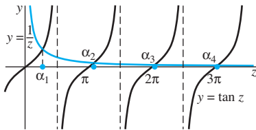
FIGURA 3.8.13. Los eigenvalores están determinados por la intersección de las gráficas de y = \tan z y y = 1/z (problema 6).
