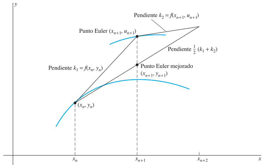
FIGURA 2.5.3. Método de Euler mejorado: promedia las pendientes de las líneas tangentes en (x_n, y_n) y (x_{n+1}, u_{n+1}) .
