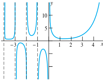
FIGURA 8.5.1. Gráfica de la función gamma extendida.
