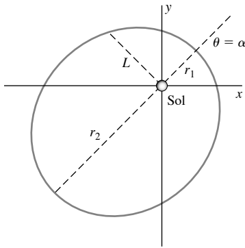
FIGURA 4.1.18. Órbita elíptica
