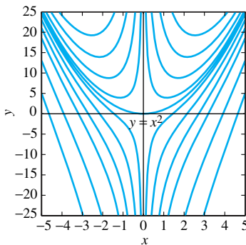
FIGURA 1.6.8. Curvas solución de la forma y = x^2 + \frac{C_1}{x} para C_1 = 0, \pm 3, \pm 10, \pm 20, \pm 35, \pm 60, \pm 100 .
