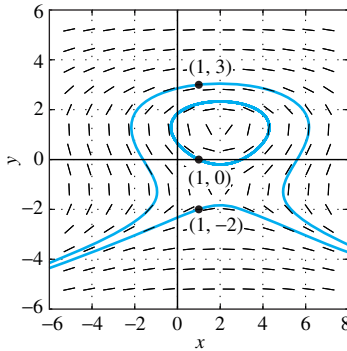
FIGURA 1.4.2. Campo de isoclinas y curvas solución para y' = (4 - 2x)/(3y^2 - 5) del ejemplo 2.
