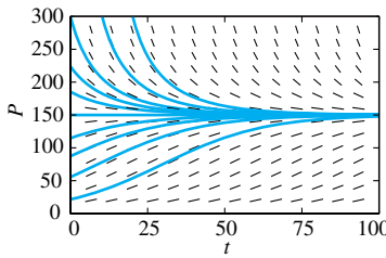
FIGURA 1.3.8. Campo de isoclinas y curvas solución P' = 0.06P - 0.0004P^2 .
