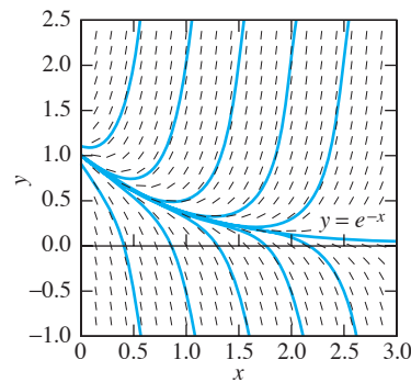
FIGURA 2.6.10. Campo de isoclinas y curvas solución para dy/dx = 5y - 6e^{-x} .
