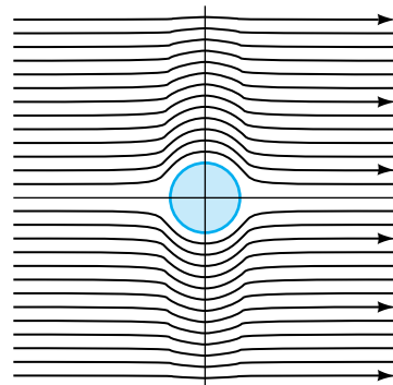
FIGURA 9.7.9. Trayectorias de un fluido ideal alrededor de un cilindro.
