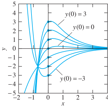
FIGURA 3.1.7. Soluciones de y'' + 3y' + 2y = 0 con la misma pendiente inicial y'(0) = 1 , pero con diferentes valores iniciales.
