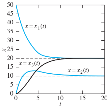
FIGURA 5.2.6. Funciones del contenido de sal del ejemplo 4.
