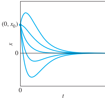
FIGURA 3.4.8. Movimiento críticamente amortiguado: x(t) = (c_1 + c_2 t)e^{-pt} con p > 0 . Las curvas solución están graficadas con la misma posición inicial x_0 para diferentes velocidades iniciales.
