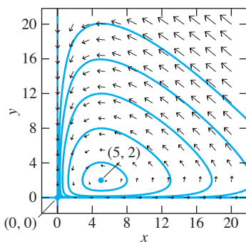
FIGURA 6.3.16. Caso en que \epsilon = 0 (problemas 18 y 19).
