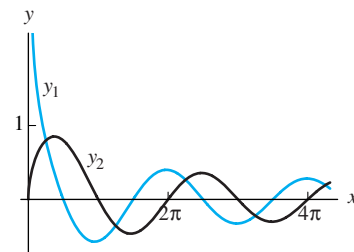
FIGURA 8.3.2. Soluciones
