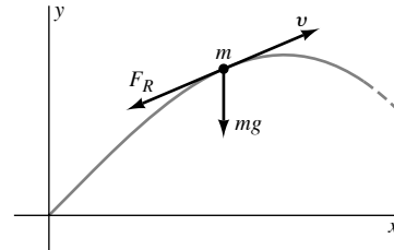
FIGURA 4.1.15. Trayectoria del proyectil del problema 30.
