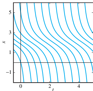
FIGURA 2.2.11. Curvas solución de la ecuación x' = x(4 - x) - h con cosecha excesiva h = 5 .
