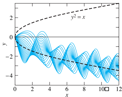
FIGURA 8.6.8. Primera trascendente de Painlevé y'' = y^2 - x , y(0) = 0 , y'(0) = -3.3, -3.1, \dots, 0.7 .
