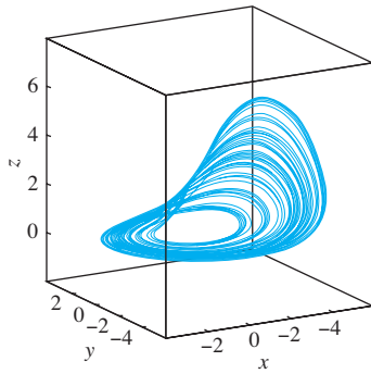
FIGURA 6.5.20. Banda de Rössler ilustrada con una trayectoria graficada con x(0) = 2 , y(0) = 0 , z(0) = 3 y 0 \leq t \leq 400 .
