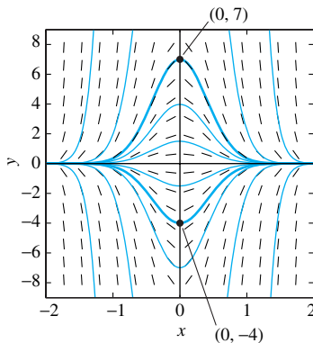
FIGURA 1.4.1. Campos de isoclinas y curvas solución para y' = -6xy en el ejemplo 1.
