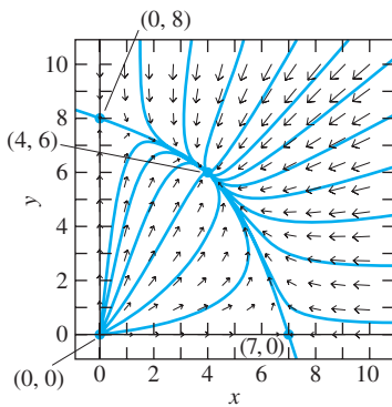
FIGURA 6.3.13. Campo direccional y plano de fase para el sistema de competencia x' = 14x - 2x^2 - xy , y' = 16y - 2y^2 - xy del ejemplo 4.
