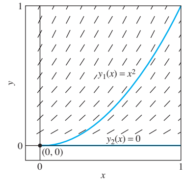
FIGURA 1.3.10. Campo direccional y dos curvas solución diferentes para el problema de valor inicial y' = 2\sqrt{y} , y(0) = 0 .
