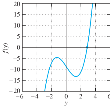
FIGURA 1.4.3. Gráfica de f(y) = y^3 - 5y - 9 .
