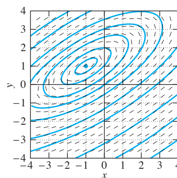
FIGURA 6.1.19. Centro estable (-1, 1)
