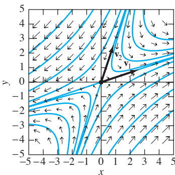
FIGURA 6.2.5. Punto silla del ejemplo 3.
