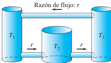
FIGURA 5.2.5. Los tres tanques de salmuera del ejemplo 4.
