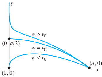
FIGURA 1.6.6. Los tres casos w < v_0 (la velocidad del avión excede la velocidad del viento); w = v_0 (velocidades iguales), y w > v_0 (el viento es mayor).
