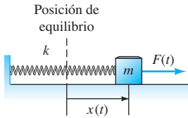
FIGURA 9.4.1. Sistema masa-resorte con una fuerza externa.
