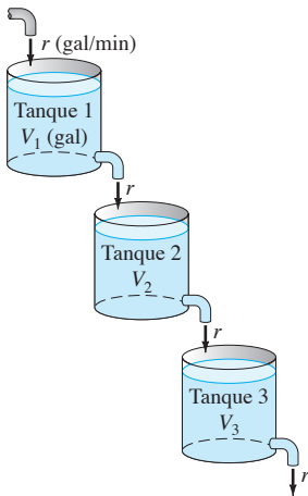
FIGURA 5.6.1. Los tres tanques de salmuera del ejemplo 2.
