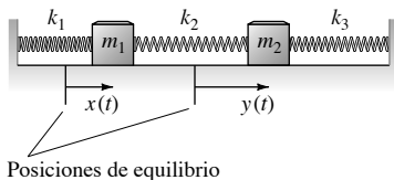
FIGURA 4.2.6. Sistema mecánico del problema 38.
