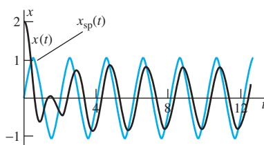
FIGURA 9.4.8. Solución periódica estacionaria x_{sp}(t) y solución amortiguada x(t) .
