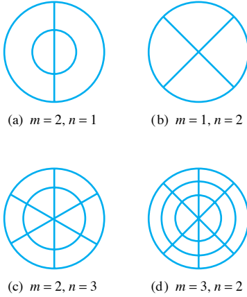
FIGURA 10.5.6. Círculos y radios nodales típicos de una membrana circular vibrando.
