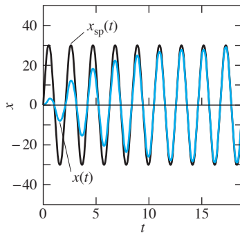
FIGURA 3.6.13. Solución x(t) = x_{tr}(t) + x_{sp}(t) y la solución periódica estacionaria x(t) = x_{sp}(t) con fuerza periódica externa F(t) = 901 \cos 3t .
