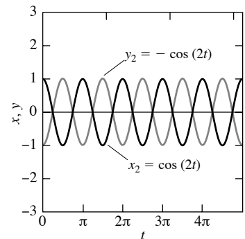
FIGURA 4.2.4. Movimiento de dos masas en direcciones opuestas, cada una con frecuencia \omega_2 = 2 .
