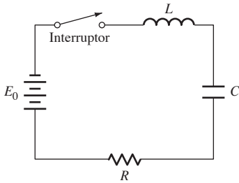
FIGURA 7.5.7. Circuito RLC en serie del ejemplo 5.
