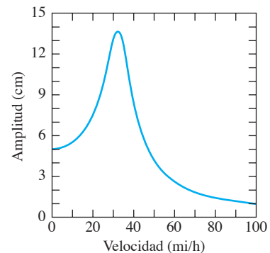
FIGURA 3.6.12. Amplitud de las vibraciones del carro en la superficie de la plataforma de lavado.
