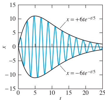
FIGURA 3.6.14. Solución x(t) = 6te^{-t/5} \sin 3t y curvas envolventes x(t) = \pm 6te^{-t/5} con fuerza oscilatoria amortiguada F(t) = 900e^{-t/5} \cos 3t .
