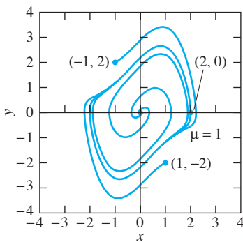
FIGURA 6.4.18. Trayectoria del plano de fase de una solución periódica de la ecuación de van der Pol con \mu = 1 , así como algunas trayectorias en espiral entrando y saliendo.
