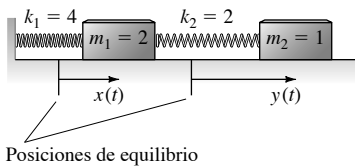
FIGURA 4.2.2. Sistema masa-resorte del ejemplo 3.
