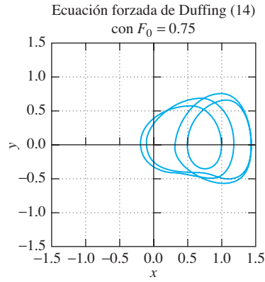
FIGURA 6.5.15(a). Respuesta de periodo 8\pi con F_0 = 0.75 : trayectoria del plano de fase.
