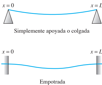
FIGURA 3.8.10. Dos maneras de soportar una viga.
