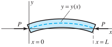
FIGURA 3.8.12. Varilla deflexionada.
