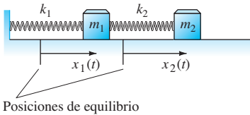
FIGURA 5.3.3. Sistema masa y resorte del ejemplo 1.
