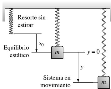
FIGURA 3.4.2. Masa suspendida desde un resorte vertical.
