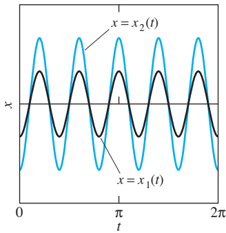
FIGURA 5.3.4. Oscilaciones en la misma dirección con frecuencia \omega_1 = 5 ; la amplitud del movimiento de la masa 2 es el doble del de la masa 1.
