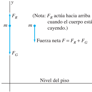
FIGURA 2.3.1. Movimiento vertical con resistencia del aire.
