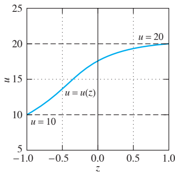
FIGURA 10.5.12. Temperatura u(z) en el punto z del eje vertical de la boya con h = 0.5 .
