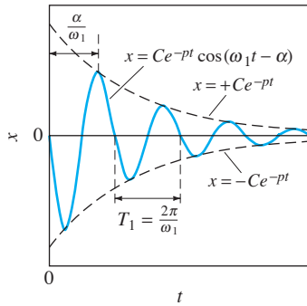
FIGURA 3.4.9. Oscilaciones subamortiguadas:
