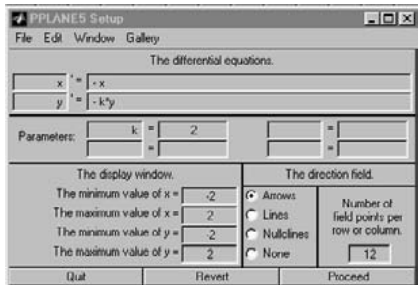
FIGURA 6.1.20. Menú de datos de entrada del programa MATLAB pplane para trazar un campo direccional y el plano de fase para el sistema x' = -x , y' = -2y (como el que se muestra en la fig. 6.1.6).
