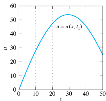
FIGURA 10.2.9. Temperaturas interiores cuando la temperatura en el lado derecho es de 25^\circ .
