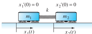
FIGURA 5.3.13. Los dos carros de ferrocarril para los problemas 16 al 19.
