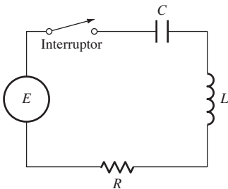
FIGURA 3.7.1. Circuito RLC en serie.
