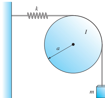
FIGURA 3.6.11. Sistema masa-resorte de la polea del problema 22.
