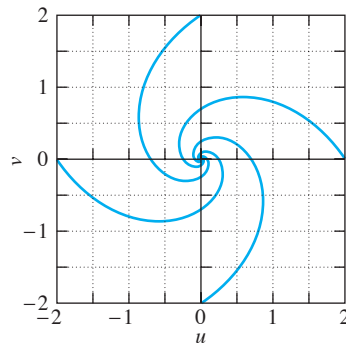
FIGURA 6.2.16. Trayectorias espirales del sistema lineal de la ecuación (21).
