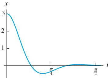
FIGURA 7.3.2. Función de la posición x(t) del ejemplo 1.
