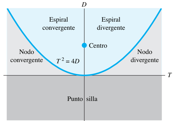
FIGURA 6.2.20. Punto crítico (0, 0) del sistema \mathbf{x}' = \mathbf{A}\mathbf{x} es:
