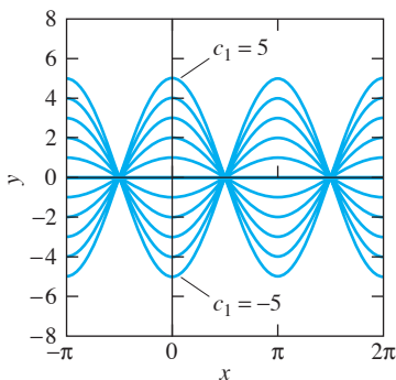
FIGURA 3.1.3. Soluciones y(x) = c_1 \cos x de y'' + y = 0 .
