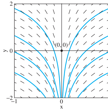
FIGURA 1.3.9. Campo direccional y curvas solución para la ecuación y' = 1/x .
