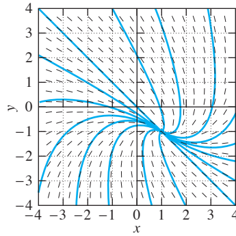
FIGURA 6.1.13. Punto espiral (1, -1) .
