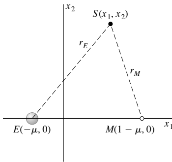
FIGURA 4.3.8. Sistema coordenado del centro de masa Tierra-Luna.
