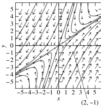
FIGURA 4.2.1. Campo direccional y curvas solución para el sistema x' = 4x - 3y , y' = 6x - 7y del ejemplo 1.
