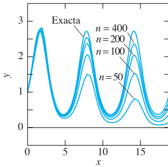
FIGURA 2.4.10. Aproximación de la solución exacta y = e^{\sin x} utilizando el método de Euler con 50, 100, 200 y 400 subintervalos.
