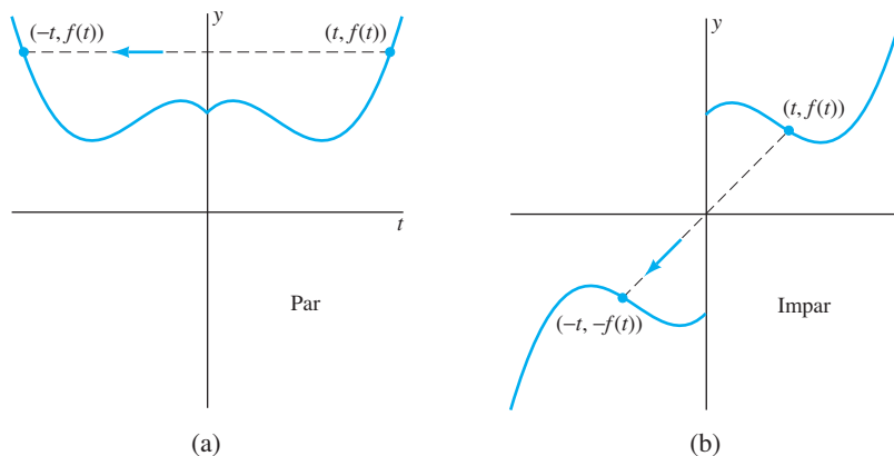
FIGURA 9.3.1. (a) Función par; (b) función impar.
