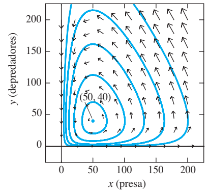
FIGURA 6.3.2. Plano de fase depredador-presa del ejemplo 2.
