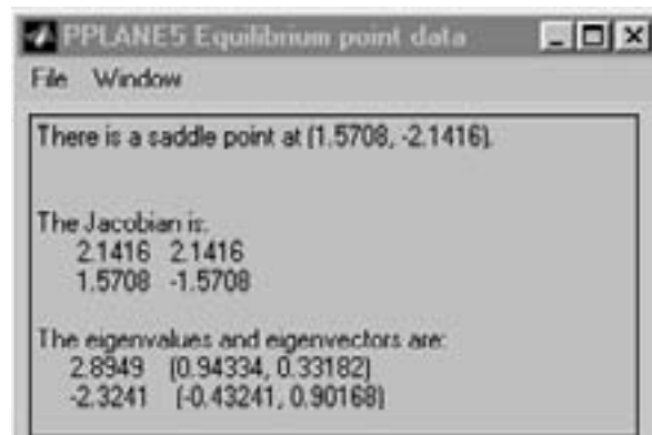
FIGURA 6.2.22. Punto silla descubierto en el cuarto cuadrante.
