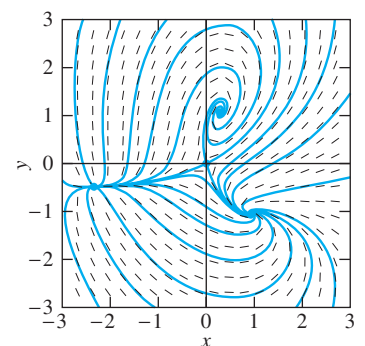
FIGURA 6.2.15. Plano de fase del sistema casi lineal de la ecuación (19).
