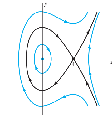
FIGURA 6.4.13. Plano de fase del problema 15.
