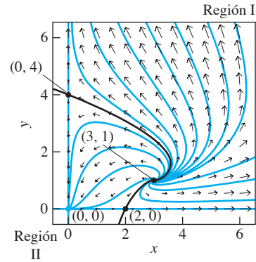
FIGURA 6.3.15. Campo direccional y plano de fase del sistema depredador-presa de los problemas 14 al 17.
