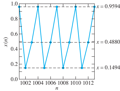
FIGURA 6.5.10. Gráfica de x(n) = x_n mostrando el ciclo de periodo 3 obtenido de iteraciones con.
