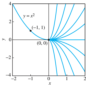
FIGURA 1.3.14. Existe una infinidad de curvas solución que pasan por el punto (-1, 1) .
