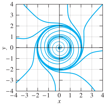
FIGURA 6.1.22. Plano de fase para el sistema correspondiente a la ecuación (5).
