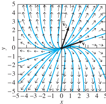
FIGURA 6.2.4. Nodo divergente impropio del ejemplo 2.
