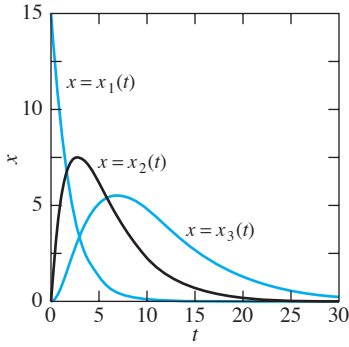
FIGURA 5.2.3. Funciones del contenido de sal en el ejemplo 2.
