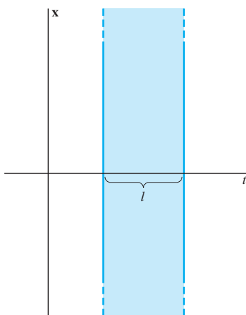
FIGURA A.1. Banda infinita en el espacio (m + 1) .
