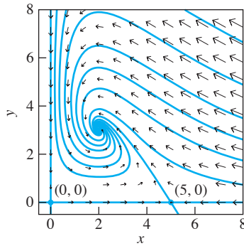
FIGURA 6.3.14. Campo direccional y plano de fase del sistema depredador-presa de los problemas 11 al 13.
