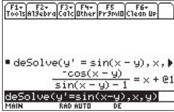
FIGURA 1.6.11. Solución implícita de y' = \sin(x - y) generada por una calculadora gráfica TI-89.
