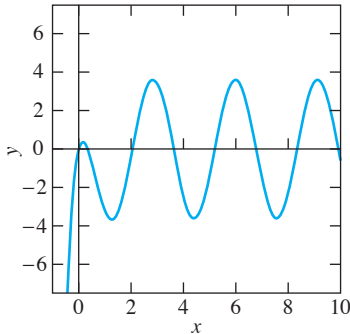
FIGURA 3.2.1. Solución particular y(x) = -3e^{-3x} + 3 \cos 2x - 2 \sin 2x .
