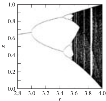
FIGURA 6.5.8. Diagrama pitchfork con 2.8 \leq r \leq 4.0 , 0 \leq x \leq 1 .
