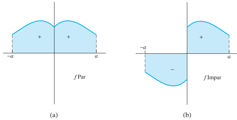
FIGURA 9.3.2. Áreas bajo las gráficas de (a) una función par y (b) una función impar.
