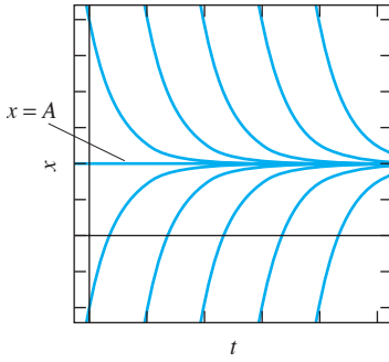
FIGURA 2.2.1. Curvas solución típicas para la ecuación de la ley de enfriamiento de Newton dx/dt = -k(x - A) .
