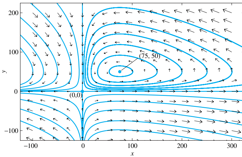
FIGURA 6.3.1. Plano de fase del sistema depredador-presa x' = 200x - 4xy , y' = -150y + 2xy con puntos críticos (0, 0) y (75, 50).
