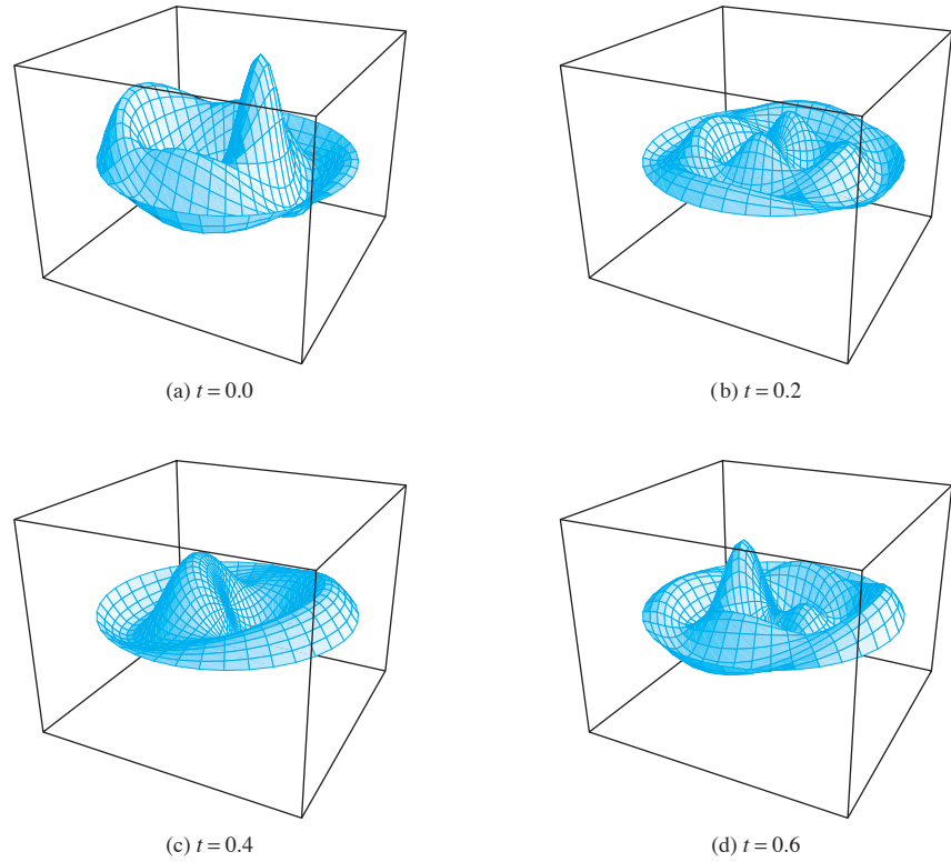
FIGURA 10.5.7. Fotografías instantáneas de la vibración de la membrana circular definida por la ecuación (54).
