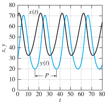
FIGURA 6.3.3. Oscilaciones periódicas de las poblaciones de presas y depredadores del ejemplo 2.
