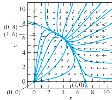
FIGURA 6.1.1. Campo direccional y plano de fase para el sistema conejos-ardillas x' = 14x - 2x^2 - xy , y' = 16y - 2y^2 - xy del ejemplo 1.
