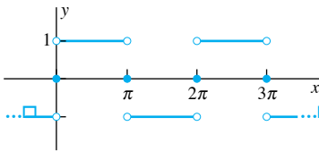
FIGURA 9.1.1. Función de onda cuadrada.
