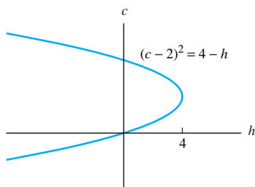
FIGURA 2.2.12. La parábola (c - 2)^2 = 4 - h representa el de diagrama de cambio de la ecuación diferencial x' = x(4 - x) - h .
