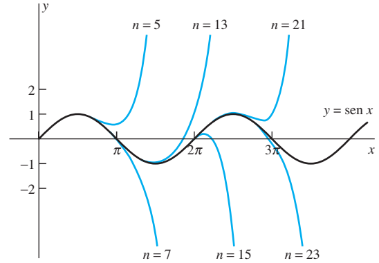
FIGURA 8.1.3. Aproximaciones polinomiales de Taylor para \sin x .
