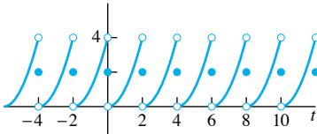
FIGURA 9.2.3. Función de periodo 2 del ejemplo 2.
