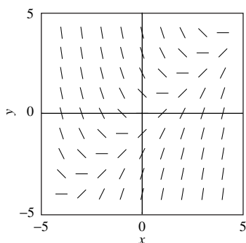
FIGURA 1.3.4. Campo de isoclinas para y' = x - y correspondientes a la tabla de pendientes de la figura 1.3.3.
