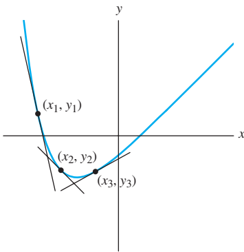
FIGURA 1.3.1. Curva solución para la ecuación diferencial y' = x - y junto con las líneas tangentes en
