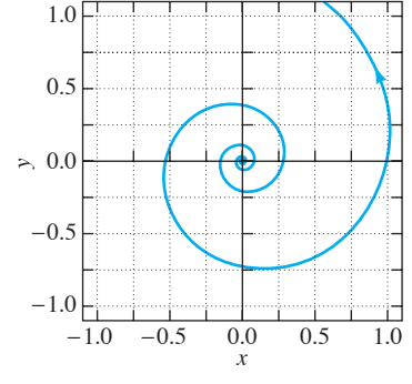
FIGURA 6.2.18 (e). Espiral inestable con \epsilon = 0.2 .
