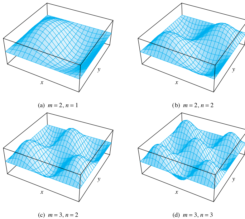
FIGURA 10.5.1. Superficies de la forma u = \sin \frac{m\pi x}{a} \sin \frac{n\pi y}{b} .
