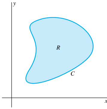
FIGURA 9.7.1. Región plana R y su curva frontera C .
