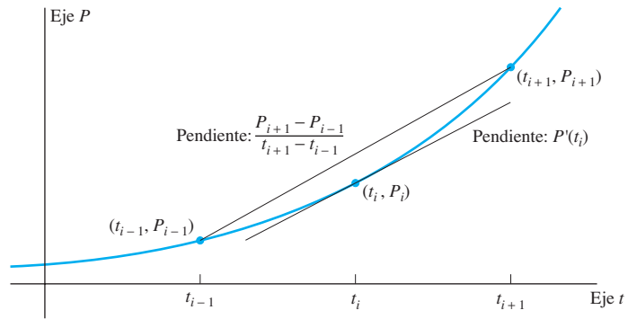
FIGURA 2.1.8. Aproximación de diferencias simétrica \frac{P_{i+1} - P_{i-1}}{t_{i+1} - t_{i-1}} para la derivada P'(t_i) .
