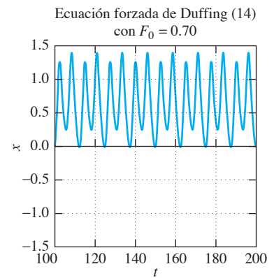
FIGURA 6.5.14(b). Respuesta de periodo 4\pi con F_0 = 0.70 : solución x(t) .
