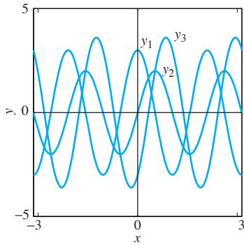
FIGURA 1.1.6. Las tres soluciones y_1(x) = 3 \cos 3x , y_2(x) = 2 \sin 3x y y_3(x) = -3 \cos 3x + 2 \sin 3x de la ecuación diferencial y'' + 9y = 0 .
