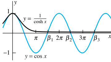
FIGURA 10.3.2. Soluciones de \cosh x \cos x = 1 .
