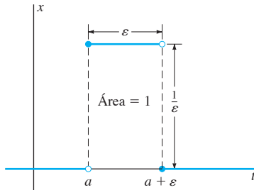
FIGURA 7.6.1. Gráfica de la función impulso d_{a,\epsilon}(t) .
