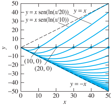
FIGURA 1.6.3. Curvas solución para xy' = y + \sqrt{x^2 - y^2} .
