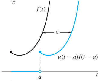
FIGURA 7.5.2. Traslación de f(t) a unidades hacia la derecha.
