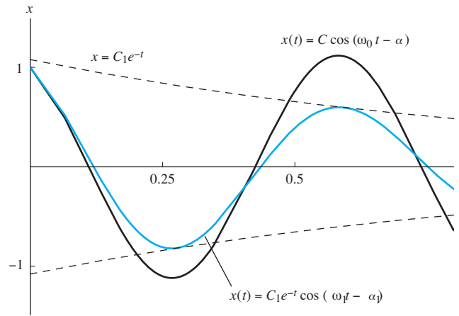
FIGURA 3.4.11. Gráficas en el intervalo 0 \leq t \leq 0.8 ilustrando el retraso adicional asociado con el amortiguamiento.
