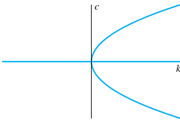
FIGURA 2.2.13. Diagrama de bifurcación para dx/dt = kx - x^3 .
