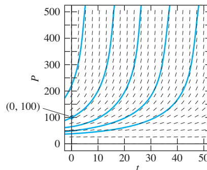
FIGURA 2.1.1. Campo de isoclinas y curvas solución para la ecuación dP/dt = (0.0005)P^2 del ejemplo 1.
