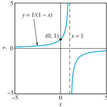
FIGURA 1.1.5. Solución de y' = y^2 definida y(x) = 1/(1 - x) .
