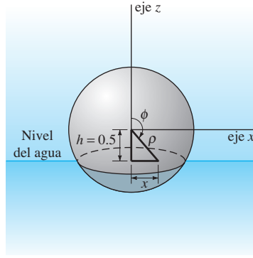
FIGURA 10.5.13. Sección transversal al nivel del agua con z = -0.5, -\frac{\sqrt{3}}{2} \leq x \leq \frac{\sqrt{3}}{2} .
