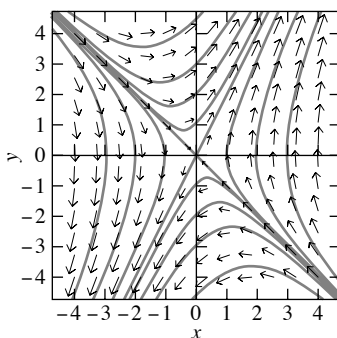
FIGURA 4.1.8. Campos direccional y curvas solución para el sistema x' = y, y' = 2x + y del ejemplo 7.
