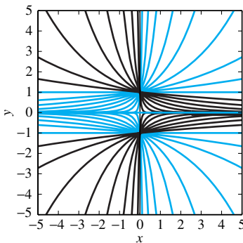
FIGURA 1.6.9. Curvas solución y = Ae^{Bx} con B = 0 y A = 0, \pm 1 son las rectas horizontales y = 0, \pm 1 . Las curvas exponenciales con B > 0 y A = \pm 1 están en gris, y aquellas con B < 0 y A = \pm 1 son negras.
