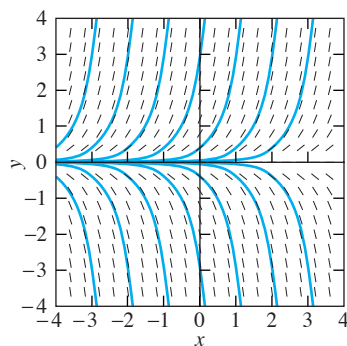
FIGURA 1.3.2(a) Campos de isoclinas y curvas solución para y' = 2y .
