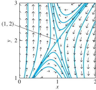
FIGURA 6.2.1. Punto silla (1, 2) para el sistema x' = 3x - x^2 - xy , y' = y + y^2 - 3xy del ejemplo 1.
