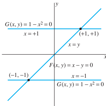
FIGURA 6.1.4. Los dos puntos críticos (-1, -1) y (+1, +1) del ejemplo 2 como la intersección de las curvas F(x, y) = x - y = 0 y G(x, y) = 1 - x^2 = 0 .
