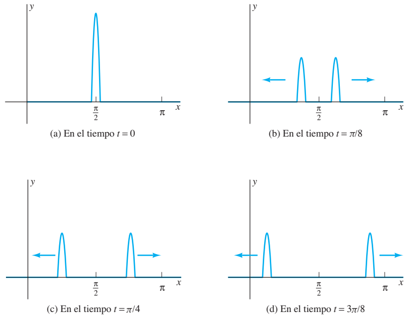
FIGURA 9.6.3. Pulso F(x) que produce dos ondas —una que se mueve a la izquierda y otra a la derecha.
