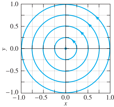
FIGURA 6.2.18 (c) Centro estable con \epsilon = 0 .
