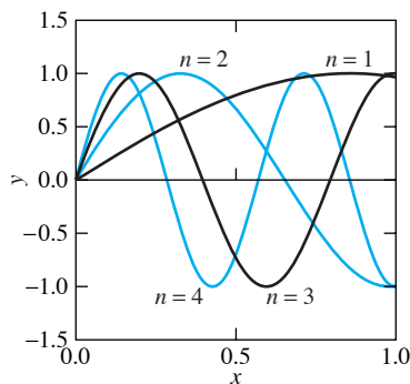
FIGURA 10.1.5. Eigenfunciones y_n(x) = \sin \beta_n x para n = 1, 2, 3, 4 .
