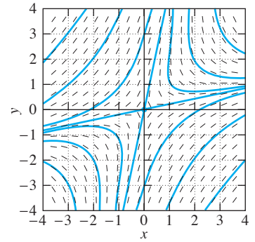
FIGURA 6.1.14. Punto silla (0, 0) .
