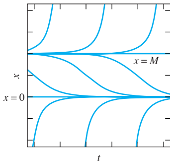
FIGURA 2.2.6. Curvas solución típicas para la ecuación explosión/extinción dx/dt = kx(x - M) .
