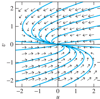
FIGURA 6.3.6. Plano de fase para el sistema lineal de la ecuación (15) correspondiente al punto crítico (28, 0).
