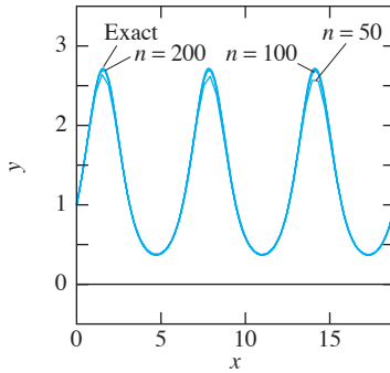
FIGURA 2.5.9. Aproximando la solución exacta y = e^{\sin x} , utilizando el método de Euler mejorado con n = 50, 100 y 200 subintervalos.
