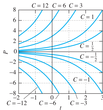
FIGURA 1.1.3. Gráficas de P(t) = Ce^{kt} con k = \ln 2 .
