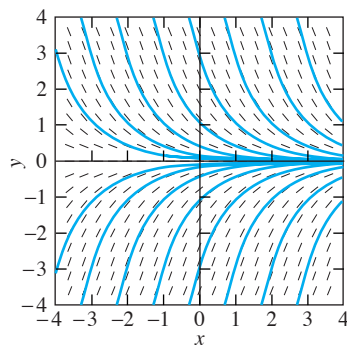
FIGURA 1.3.2(c) Campos de isoclinas y curvas solución para y' = -y .
