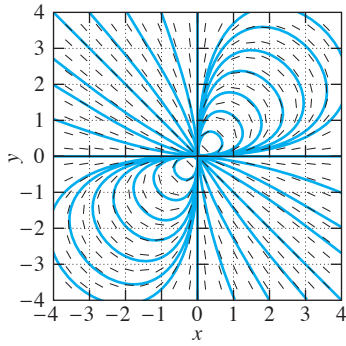
FIGURA 6.1.21. Plano de fase para el sistema de la ecuación (4).
