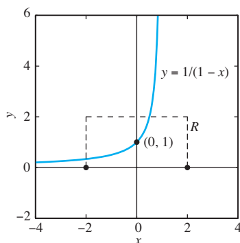
FIGURA 1.3.12. La curva solución que pasa por el punto inicial (0, 1) abandona el rectángulo R antes de que alcance el lado derecho R .
