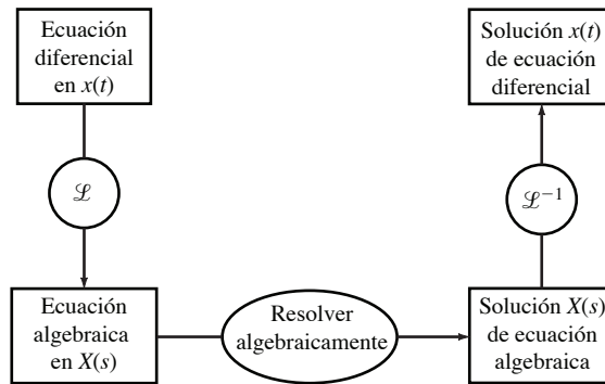
FIGURA 7.2.4. Uso de la transformada de Laplace para resolver un problema con valores iniciales.
