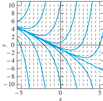
FIGURA 1.5.8. Campo de isoclinas y curvas solución para y' = x + y .
