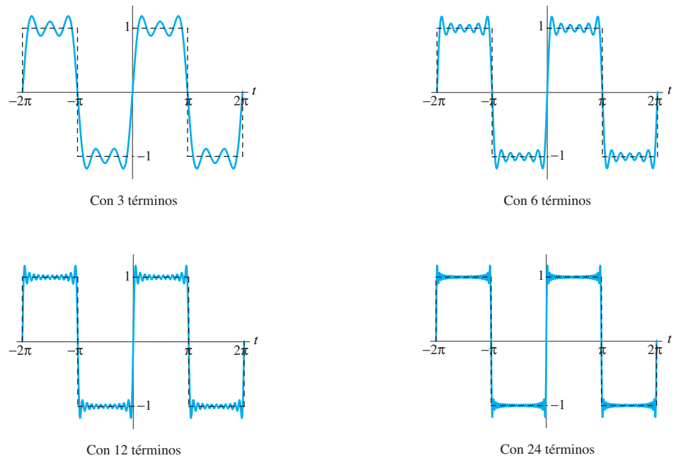
FIGURA 9.1.3. Gráficas de las sumas parciales de la serie de Fourier de la función de onda cuadrada (ej. 1) para N = 3, 6, 12 y 24 términos.
