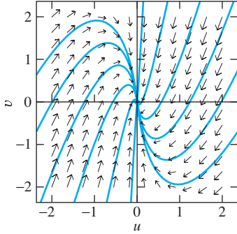
FIGURA 6.3.5. Plano de fase para el sistema lineal de la ecuación (13) correspondiente al punto crítico (0, 32).
