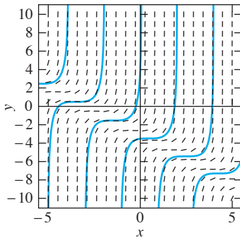
FIGURA 1.6.1. Campo de isoclinas y curvas solución para y' = (x + y + 3)^2 .
