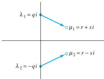
FIGURA 6.2.10. Efectos de la perturbación de las raíces imaginarias puras.
