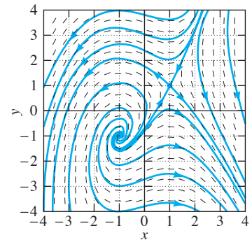
FIGURA 6.1.3. Imagen del plano de fase para el sistema en la ecuación (7).
