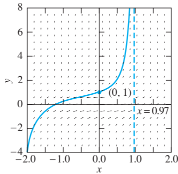
FIGURA 2.6.3. Solución de dy/dx = x^2 + y^2 , y(0) = 1 .
