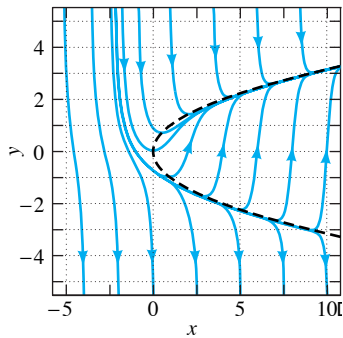
FIGURA 8.6.7. Curvas solución
