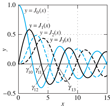
FIGURA 10.5.5. Gráficas y ceros iniciales de las primeras funciones de Bessel.
