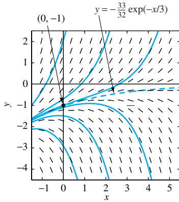
FIGURA 1.5.1. Campo de isoclinas y curvas solución para y' = y + \frac{11}{8}e^{-x/3} .
