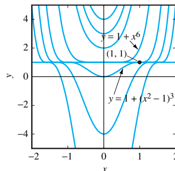
FIGURA 1.4.6. Curvas solución general y curva solución singular para y' = 6x(y - 1)^{2/3} .
