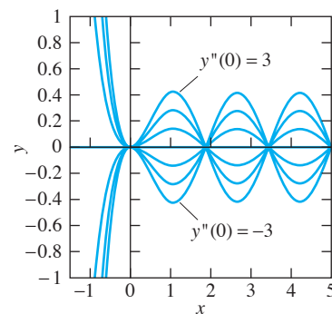
FIGURA 3.2.4. Soluciones de y^{(3)} + 3y'' + 4y' + 12y = 0 con y'(0) = y''(0) = 0 , pero con valores diferentes para y''(0) .
