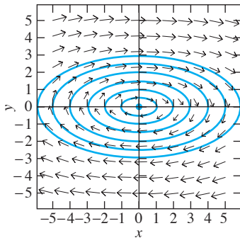
FIGURA 6.1.8. Campo direccional y trayectorias elípticas para el sistema x' = y , y' = -\frac{1}{4}x . El origen es un centro estable.
