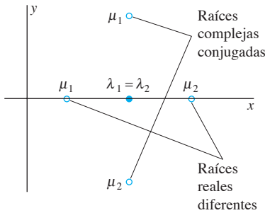
FIGURA 6.2.11. Efectos de perturbaciones de raíces reales iguales.
