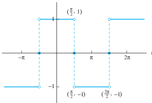
FIGURA 9.3.9. Función de onda cuadrada par de periodo 2\pi .
