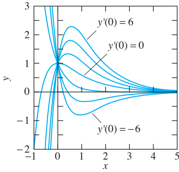
FIGURA 3.1.6. Soluciones de y'' + 3y' + 2y = 0 con el mismo valor inicial y(0) = 1 , pero con pendientes iniciales diferentes.
