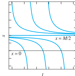
FIGURA 2.2.14. Curvas solución para una población logística con cosecha 4h = kM^2 .
