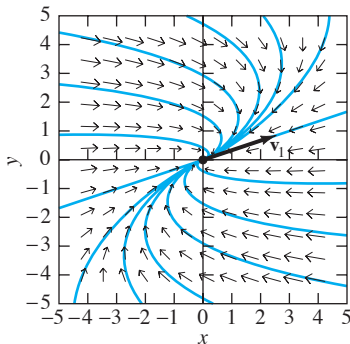
FIGURA 6.2.6. Nodo convergente impropio del ejemplo 4.
