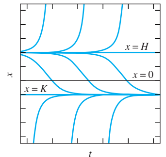
FIGURA 2.2.15. Curvas solución por cosecha en una población de lagartos.
