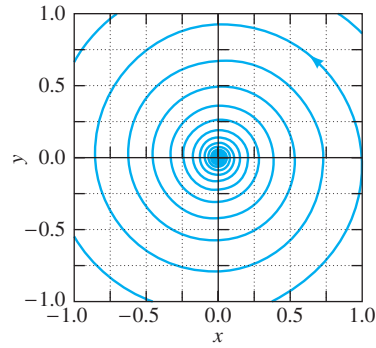
FIGURA 6.2.18 (b). Espiral estable con \epsilon = -0.05 .
