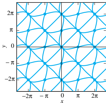
FIGURA 6.4.11. Trayectorias del sistema en el problema 2.
