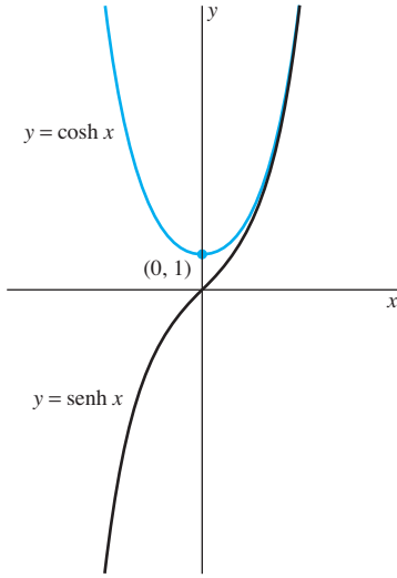
FIGURA 3.8.3. Gráficas de seno y coseno hiperbólicos.
