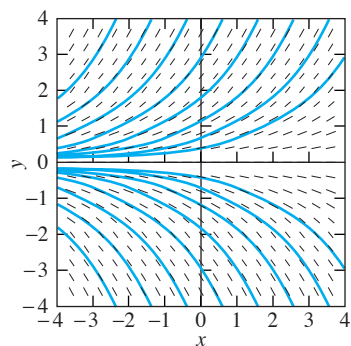
FIGURA 1.3.2(b) Campos de isoclinas y curvas solución para y' = (0.5)y .
