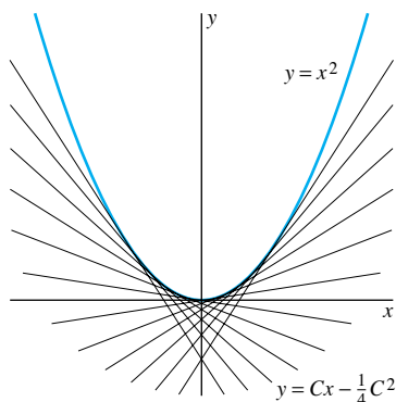
FIGURA 1.6.10. Solución de la ecuación de Clairaut del problema 67. La línea recta “típica” con ecuación y = Cx - \frac{1}{4}C^2 es tangente a la parábola en el punto (\frac{1}{2}C, \frac{1}{4}C^2) .
