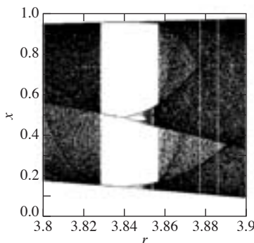
FIGURA 6.5.9. Diagrama pitchfork con 3.8 \leq r \leq 3.9 , 0 \leq x \leq 1 .
