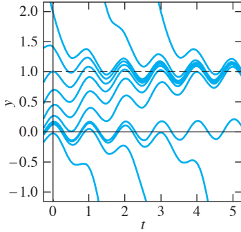
FIGURA 2.5.12. Curvas solución de dy/dt = y(1 - y) - \sin 2\pi t .
