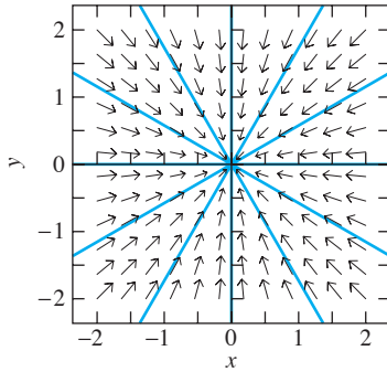
FIGURA 6.1.5. Nodo propio: las trayectorias se acercan al origen, por tanto es un nodo convergente.
