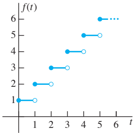
FIGURA 7.2.8. Gráfica de la función escalera unitaria del ejemplo 7.
