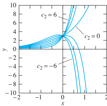
FIGURA 3.1.8. Diferentes soluciones y(x) = 3e^x + c_2 x e^x de y'' - 2y' + y = 0 con el mismo valor inicial y(0) = 3 .
