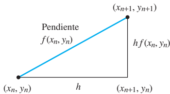
FIGURA 2.4.2. El paso de (x_n, y_n) a (x_{n+1}, y_{n+1}) .
