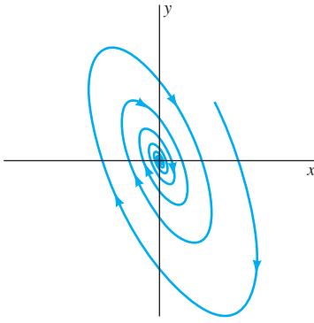
FIGURA 6.1.10. Punto espiral estable y una trayectoria hacia éste.
