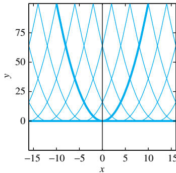
FIGURA 1.4.5. Curvas solución general y = (x - C)^2 y curva solución singular y = 0 de la ecuación diferencial (y')^2 = 4y .
