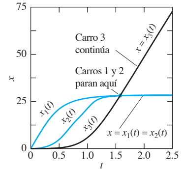
FIGURA 5.3.8. Funciones de la posición de los tres carros de ferrocarril del ejemplo 2.
