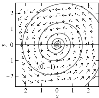
FIGURA 4.1.9. Campo direccional y curvas solución para el sistema x' = -y , y' = (1.01)x - (0.2)y del ejemplo 8.
