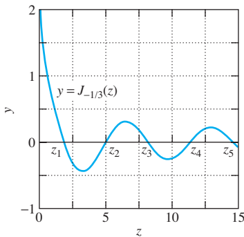
FIGURA 8.6.2. Gráfica de J_{-1/3}(z) .
