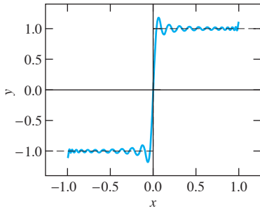
FIGURA 10.5.9. Gráfica de la suma parcial con 25 términos de la serie de onda cuadrada de la ecuación (66).
