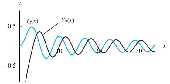
FIGURA 8.5.5. Gráficas de las funciones de Bessel J_2(x) y Y_2(x) .
