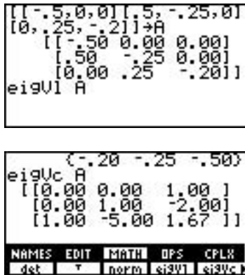
FIGURA 5.2.9. Cálculo de los eigenvalores y eigenvectores de la matriz \mathbf{A} en TI-86.
