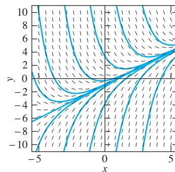
FIGURA 1.5.7. Campo de isoclinas y curvas solución para y' = x - y .
