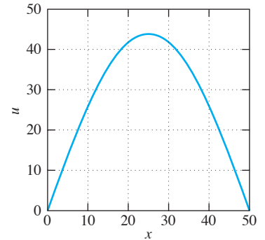
FIGURA 9.5.8. Gráfica de u(x, 1800) que proporciona las temperaturas de la barra después de 30 min.
