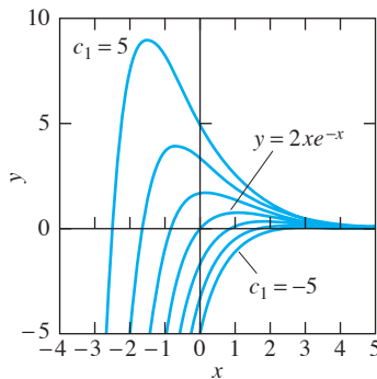
FIGURA 3.1.10. Soluciones y(x) = c_1e^{-x} + 2xe^{-x} de y'' + 2y' + y = 0 con diferentes valores de c_1 .
