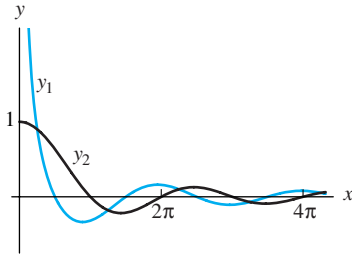
FIGURA 8.3.1. Soluciones y_1(x) = \frac{\cos x}{x} y y_2(x) = \frac{\sin x}{x} del ejemplo 6.
