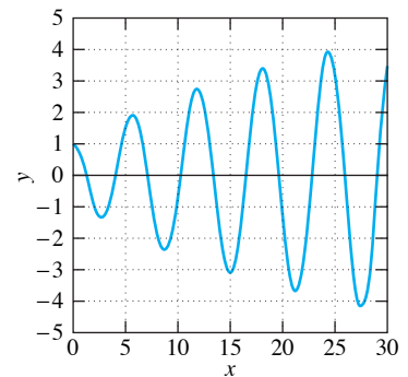
FIGURA 10.4.13. Gráfica y = J_0(x) - xJ'_0(x) .
