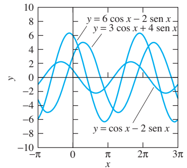
FIGURA 3.1.5. Soluciones de y'' + y = 0 con c_1 y c_2 , ambas diferentes de cero.
