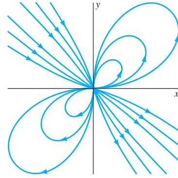
FIGURA 6.2.19. Trayectorias del sistema de la ecuación (22).
