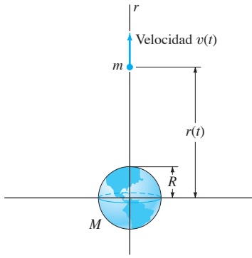
FIGURA 2.3.4. Masa m a gran distancia de la Tierra.
