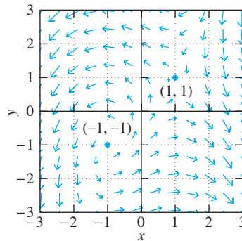
FIGURA 6.1.2. Campo direccional para el sistema en la ecuación (7).
