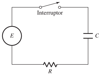
FIGURA 3.7.8. Circuito para los problemas 7 al 10.
