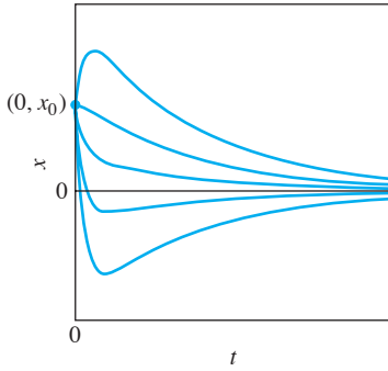
FIGURA 3.4.7. Movimiento sobreamortiguado: x(t) = c_1 e^{r_1 t} + c_2 e^{r_2 t} con r_1 < 0 y r_2 < 0 . Las curvas solución están graficadas con la misma posición inicial x_0 para diferentes velocidades iniciales.
