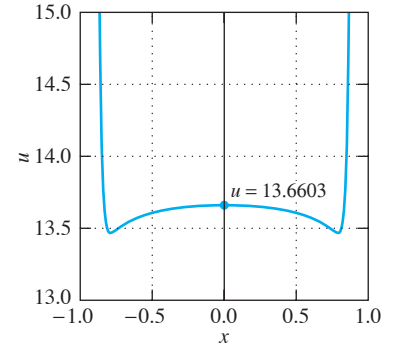
FIGURA 10.5.14. Temperatura u(x) en la sección transversal de la boya al nivel del agua con h = 0.5 .
