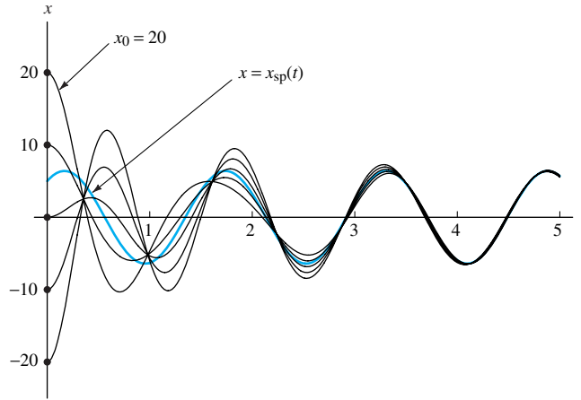
FIGURA 3.6.8. Soluciones del problema de valores iniciales en (24) con x_0 = -20, -10, 0, 10 y 20 .
