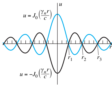
FIGURA 10.4.6. Sección transversal de la membrana circular vibrando.
