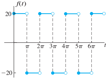
FIGURA 7.5.11. Gráfica de la función de la fuerza externa del ejemplo 8.
