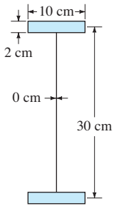
FIGURA 10.3.3. Viga idealizada con forma de I .
