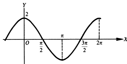
(d) y = 2 \cos x
