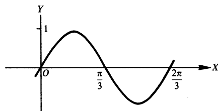
(b) y = \sin 3x
