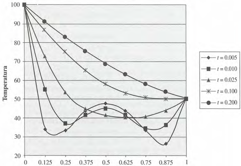
Figura 8.10 Gráfica de la distribución de temperatura a diferentes tiempos.
