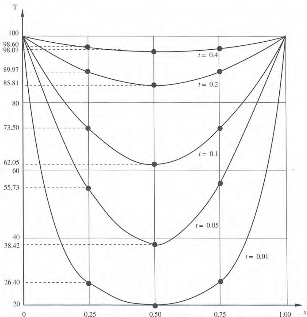
Figura 8.8 Distribución de la temperatura en la barra a diferentes tiempos.
