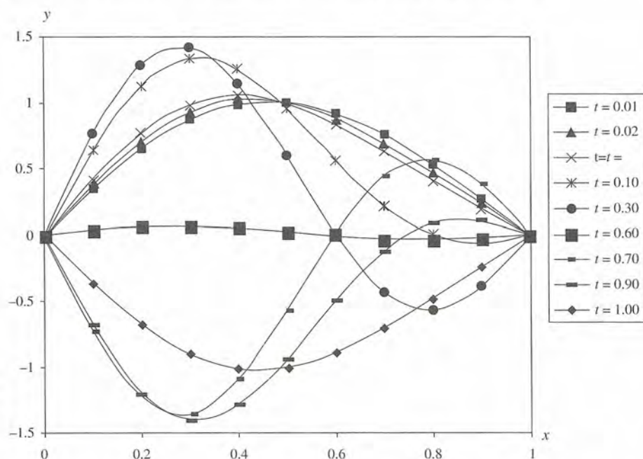
Figura 8.21 Gráfica de las posiciones de la cuerda a diferentes tiempos.
