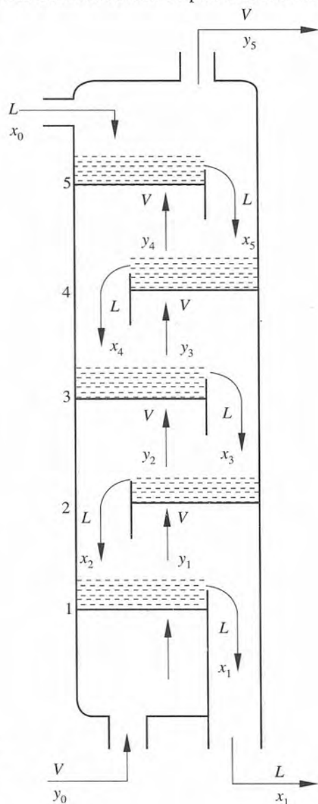
Fig. 3.13 Columna de absorción de cinco platos.
