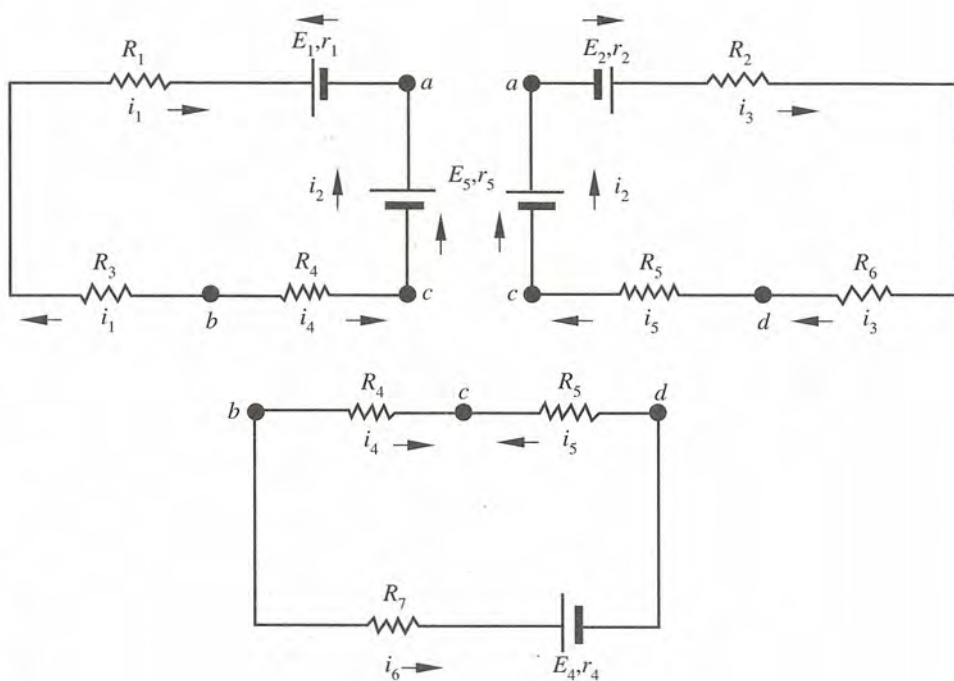
Figura 3.16 Circuito de la figura 3.15 cortado en mallas.
