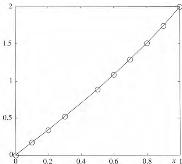
Figura 7.14 Solución gráfica del PVF.
