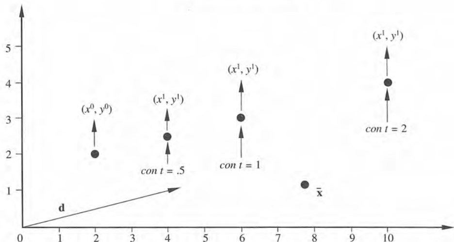
Figura 4.11 Influencia de t en el vector \mathbf{x}^{(k+1)} .
