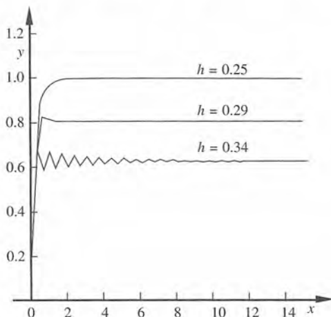
Figura 7.26 Soluciones numéricas del PVI (1) con diferentes tamaños de paso.
