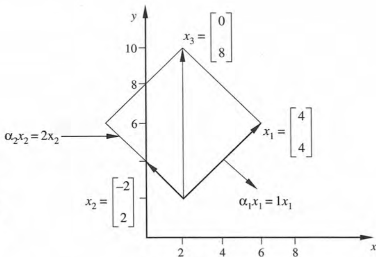
Figura 3.3 Interpretación geométrica de independencia lineal en el plano.
