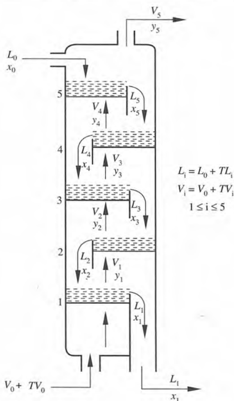
Figura 4.16 Columna de absorción de cinco platos.
