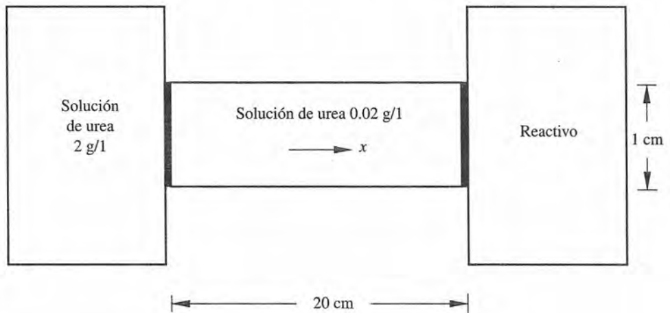
Figura 8.30 Difusión de urea en una solución.
