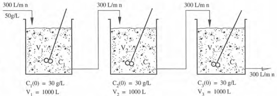
Figura 7.33 Arreglo de tres tanques interconectados.
