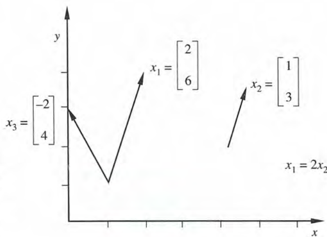
Figura 3.4 Interpretación geométrica de dependencia lineal en el plano.
