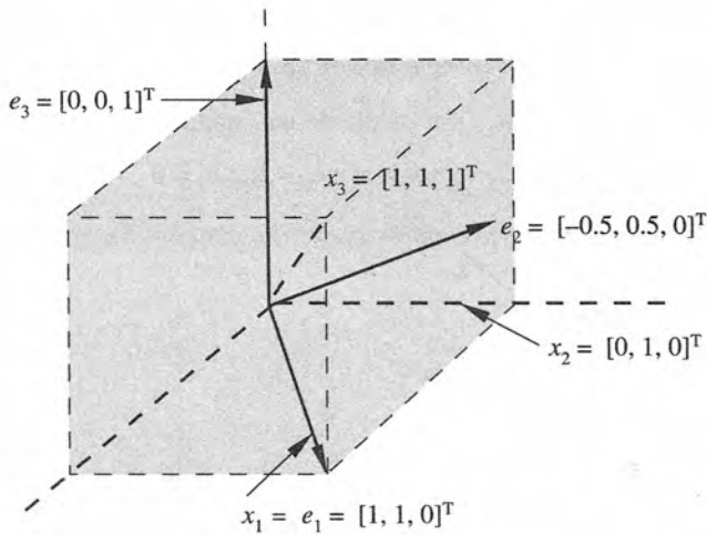
Figura 3.8 Ortogonalización en el espacio.
