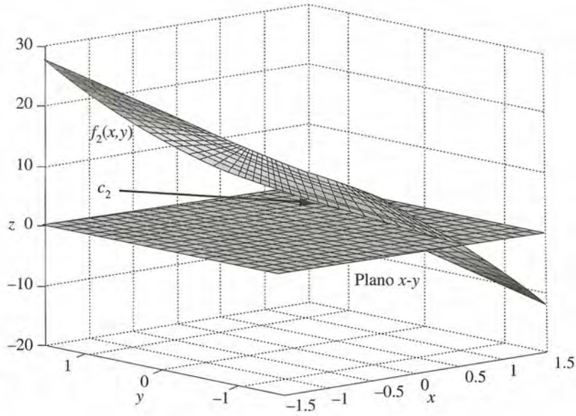
Figura 4.2 Intersección de la superficie f_2(x, y) con el plano x-y .
