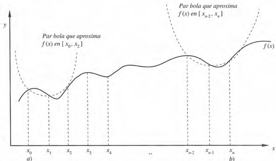
Figura 6.6 Integración por método de Simpson compuesto.
