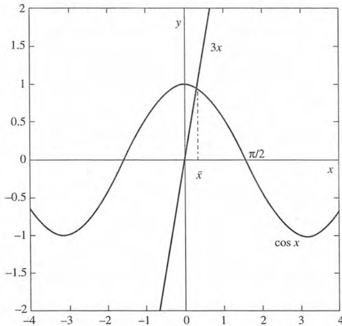
Figura 2.1 Gráfica de \cos x y de 3x .
