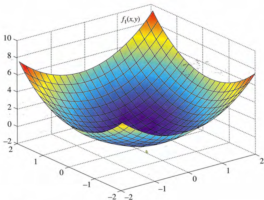
Figura 4.4 Gráfica de la superficie f_1(x, y) .
